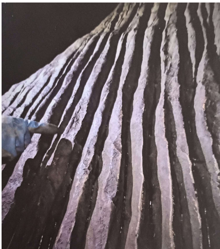
Slika 6-4 Prikaz škrapa u špiljskom sustavu Đulin ponor – Medvedica(Kovač Konrad i dr., 2022)
