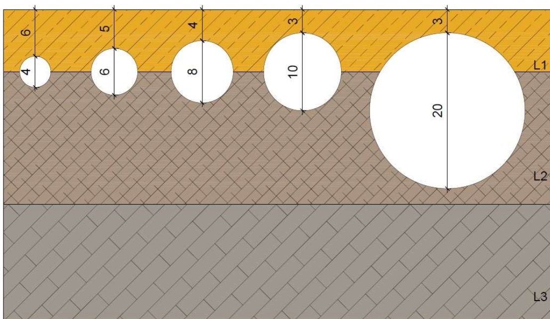
Slika 5-12. Geometrije Modela 2
