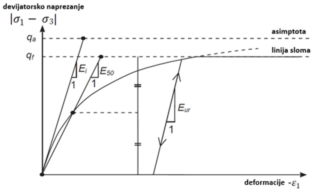
Slika 5-3. Hiperbolički odnos naprežanja i deformacija u primarnom opterećenju za standardno drenirano troosno ispitivanje (PLAXIS, 2016)
