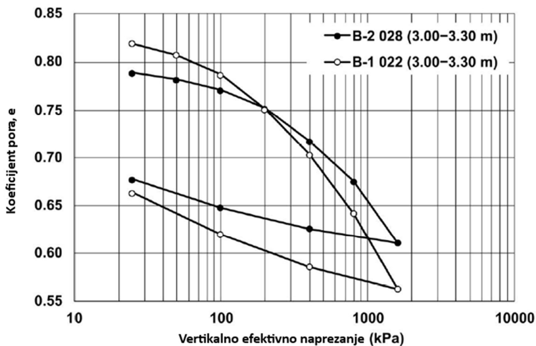
Slika 4-7. Rezultati edometarskog ispitivanja (Tomic i dr., 2021)
