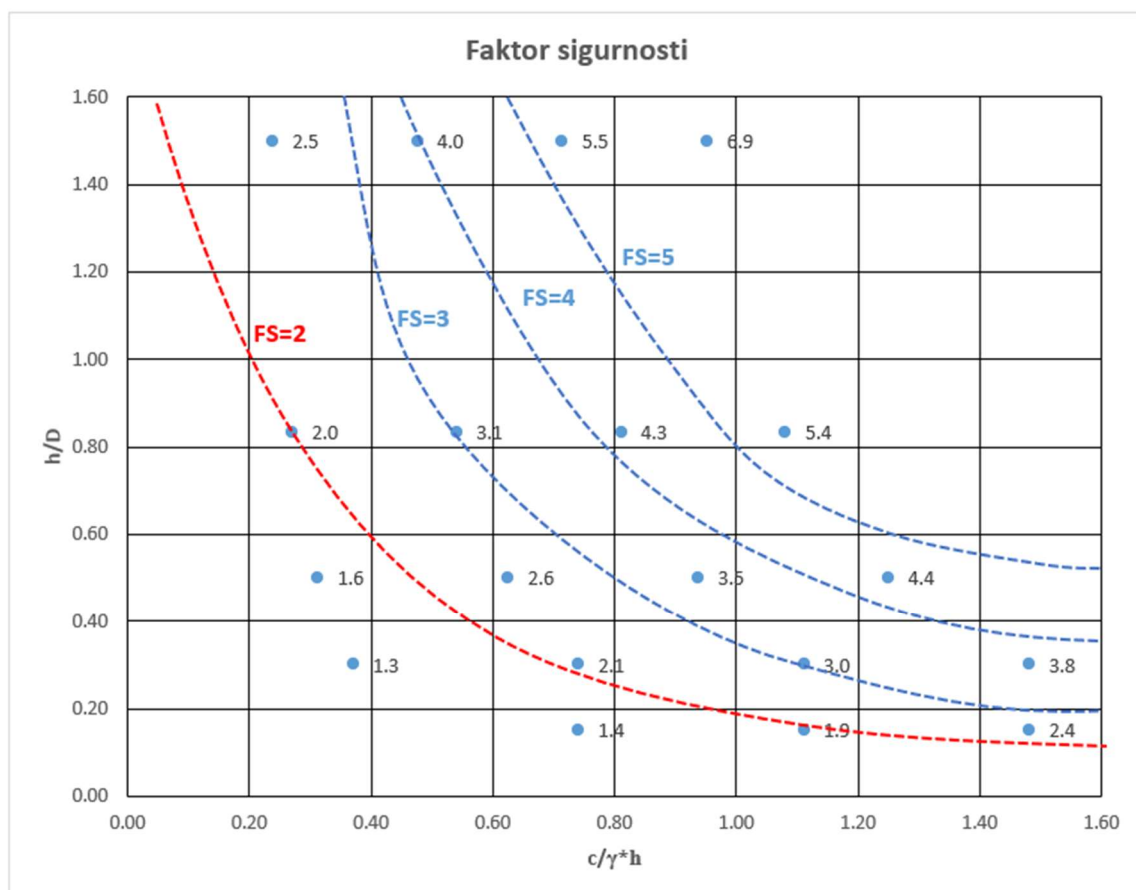
Slika 5-17. Ovisnost faktora sigurnosti o geometrijskim uvjetima i stanju naprezanja
