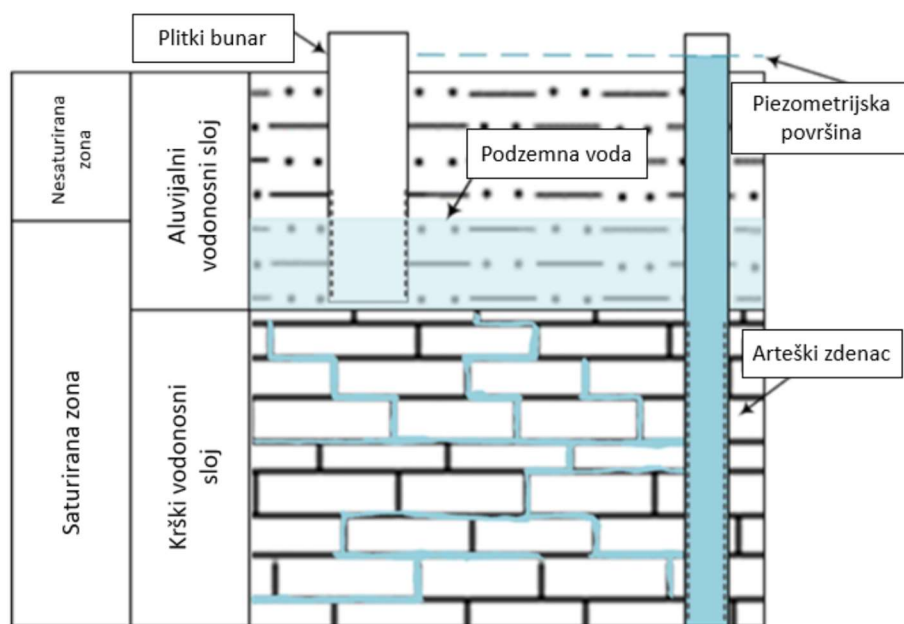
Slika 3-10. Pretpostavka piezometarske razine krškog i aluvijalnog vodonosnika (Tomic i dr., 2021)
