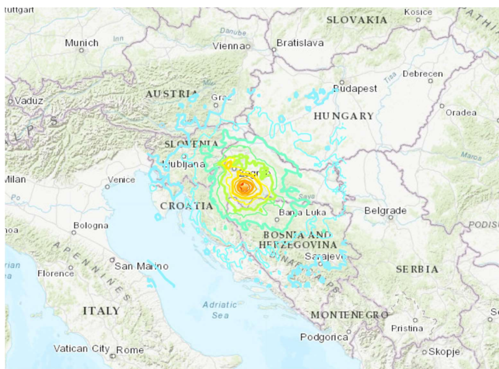
Slika 3-1. Karta podrhtavanja površine tla za vrijeme glavnog potresa u Petrinji izraženo vrijednostima horizontalnih vršnih ubrzanja tla u postocima gravitacijskog ubrzanja (Earthquake, 2022)
