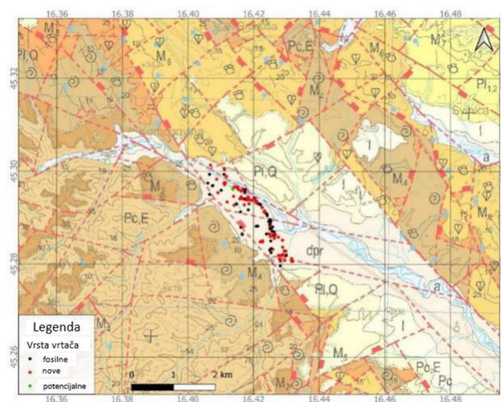
Slika 3-6. OGK Hrvatske s označenim vrtačama (Tomic i dr., 2021)
