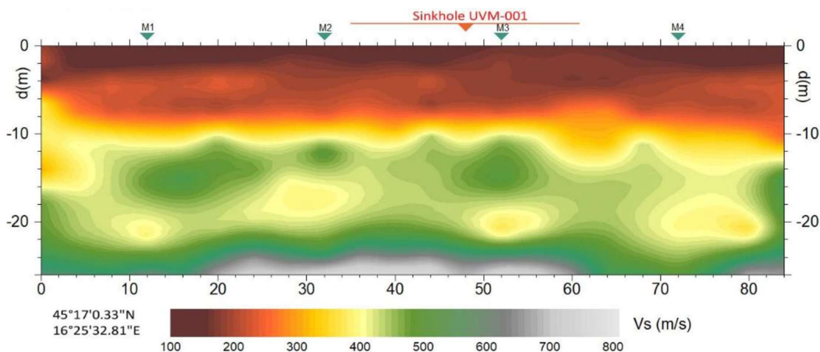
Slika 4-6. MASW profil ispod najveće vrtače (Tomic i dr., 2021)
