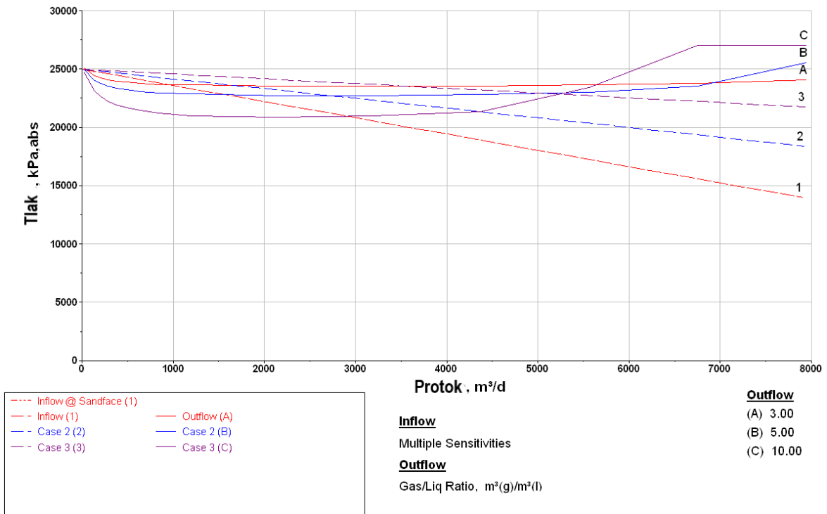
Slika 6-6. Graf analize osjetljivosti eruptivne proizvodnje bušotine Zb - 1 jug, varijanta E (Vlastita izrada prema AZU, 2024)
