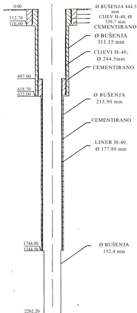
Slika 6-1. Konfiguracija bušotine Savica-1 (Geotehnika – Zagreb, 1986)
