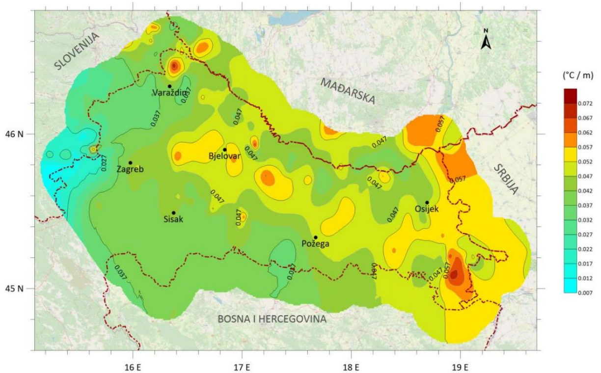
Slika 6-2. Nova karta geotermalnih gradijenata na području kontinentalne Hrvatske (Macenić, 2020)
