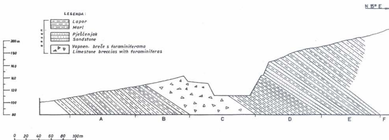
Sl.1. Geološki profil kroz ležište "Partizan"
