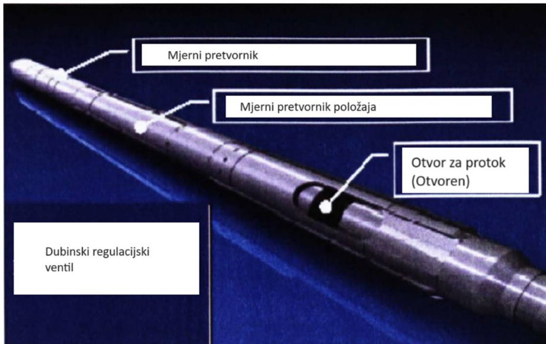
Slika 2-22. Dubinski regulacijski ventil (ICV) (Reyes i Arias, 2004)
