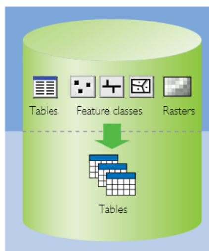
Slika 2-7. Razine geoprostorne baze podataka (Zeiler & Murphy, 2010)
