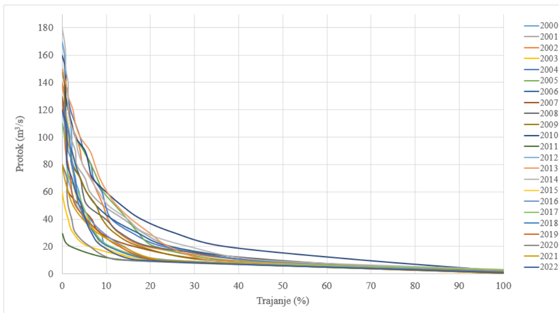
Slika 4.9. Krivulja trajanja protoka rijeke Tounjčice
