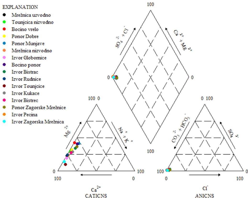
Slika 5.26. Piperov dijagram
