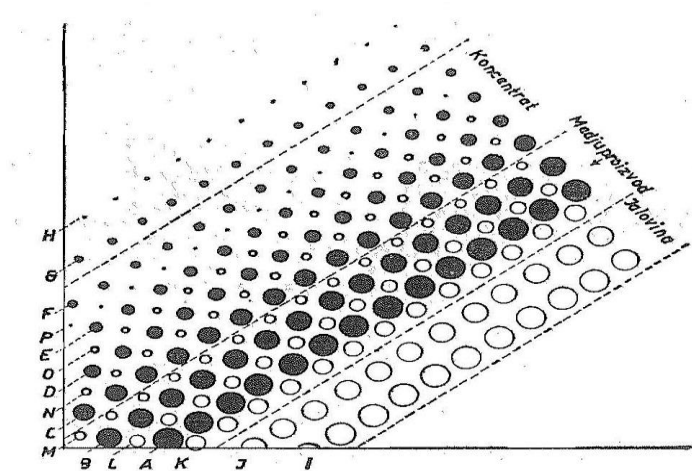
Slika 5-3. Idealan raspored zrna na ploči koncentracijskog stola (Lešić i Marković 1968).
