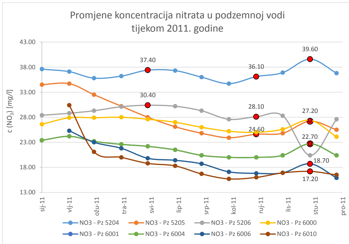
Slika 6.3.5. Mjesečne koncentracije nitrata u podzemnoj vodi u 2011. godini iz 8 piezometara unutar istraživanih područja s naznačenim povišenim vrijednostima koncentracija nitrata
