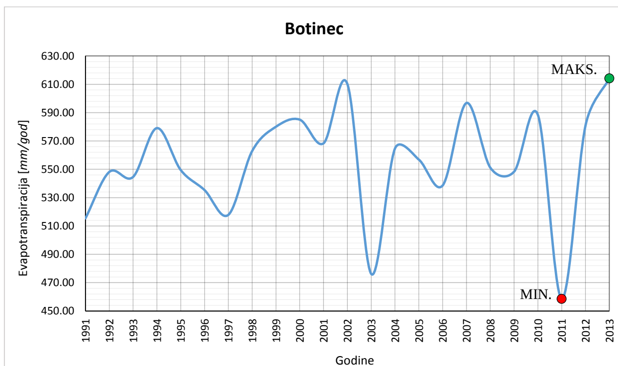
Slika 2.3.5. Evapotranspiracija u vremenskom razdoblju od 1991. do 2013. godine izračunata na temelju podataka mjerenih na meteorološkoj stanici Botinec s naznačenim maksimalnim i minimalnim vrijednostima evapotranspiracije
