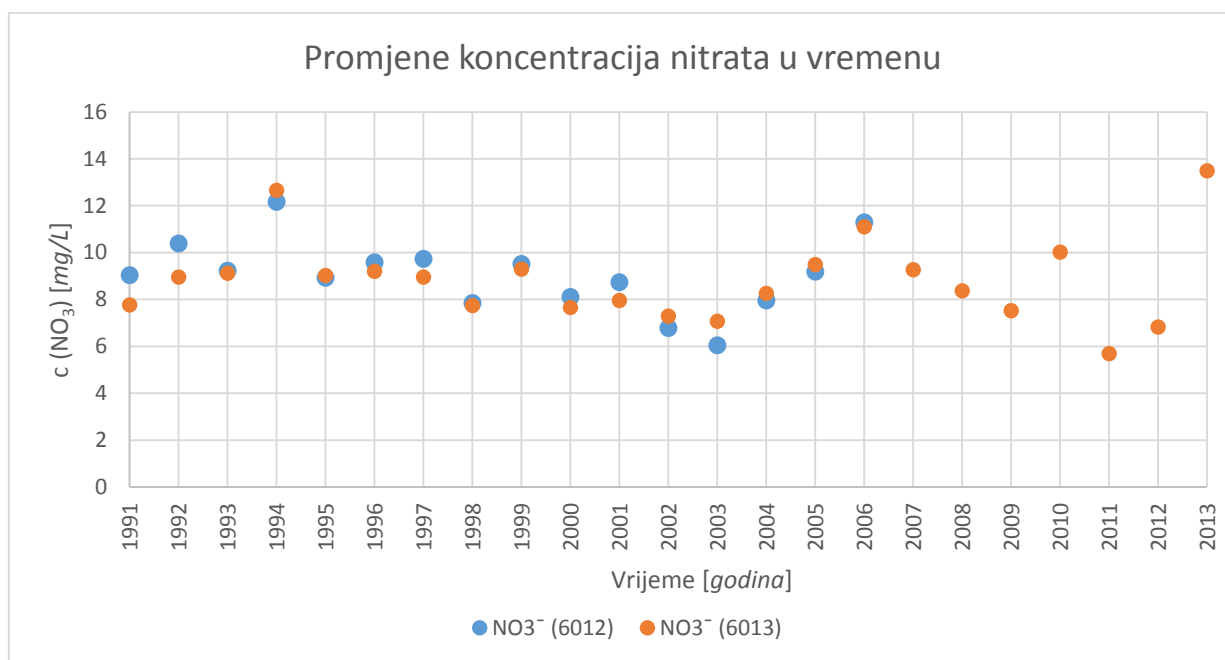
Slika 6.1.3. Promjene koncentracija nitrata u podzemnoj vodi u vremenu na piezometrima 6012 i 6013
