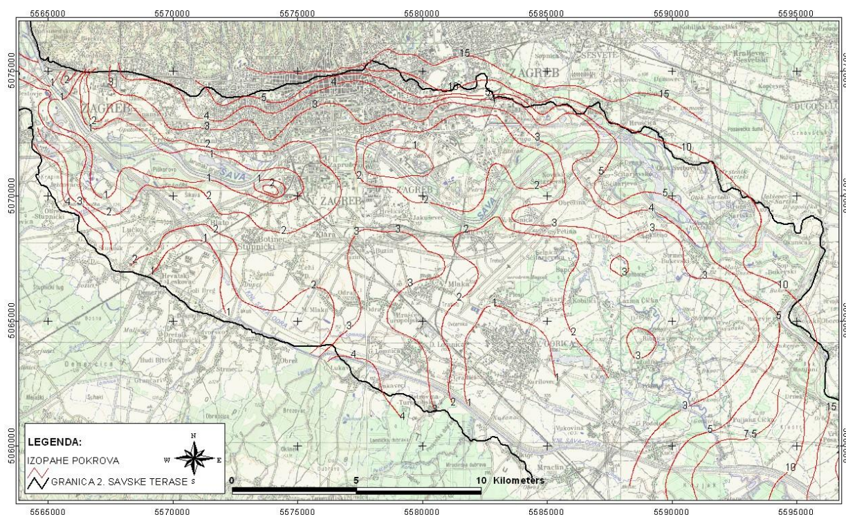
Slika 2.2.2. Izopahe pokrova vodonosnog sustava (Bačani i Posavec, 2009.)
