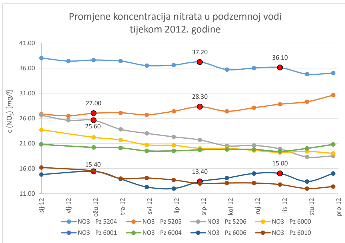
Slika 6.3.6. Mjesečne koncentracije nitrata u podzemnoj vodi u 2012. godini iz 8 piezometara unutar istraživanih područja s naznačenim povišenim vrijednostima koncentracija nitrata
