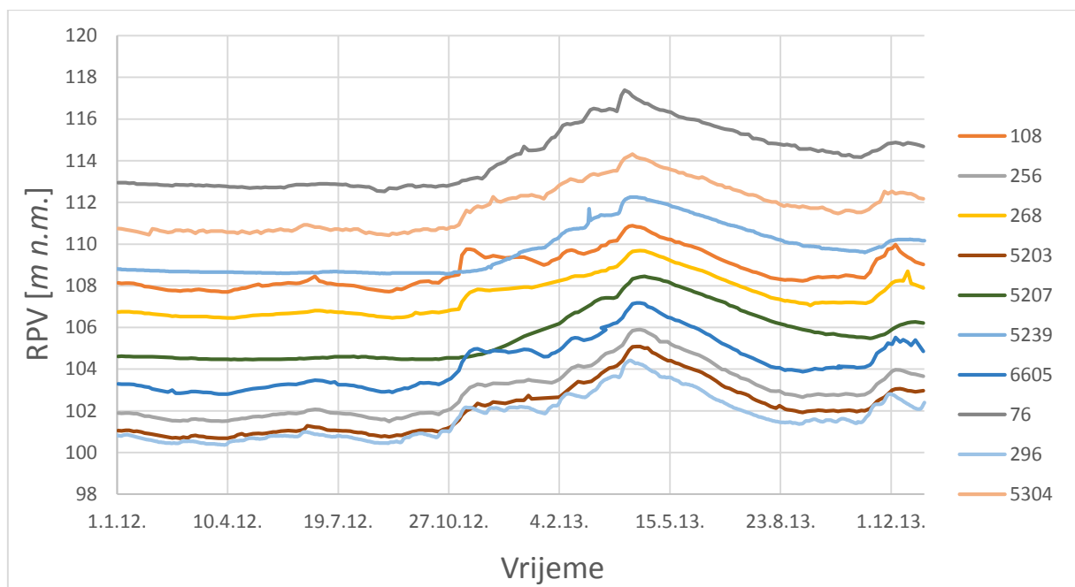
Slika 2.3.3. Promjene razina podzemne vode za vremensko razdoblje od 1.1.2012. do 31.12.2013. godine mjerene na piezometrima unutar istraživanog područja
