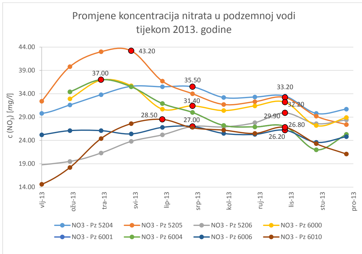
Slika 6.3.7. Mjesečne koncentracije nitrata u podzemnoj vodi u 2013. godini iz 8 piezometara unutar istraživanih područja s naznačenim povišenim vrijednostima koncentracija nitrata
