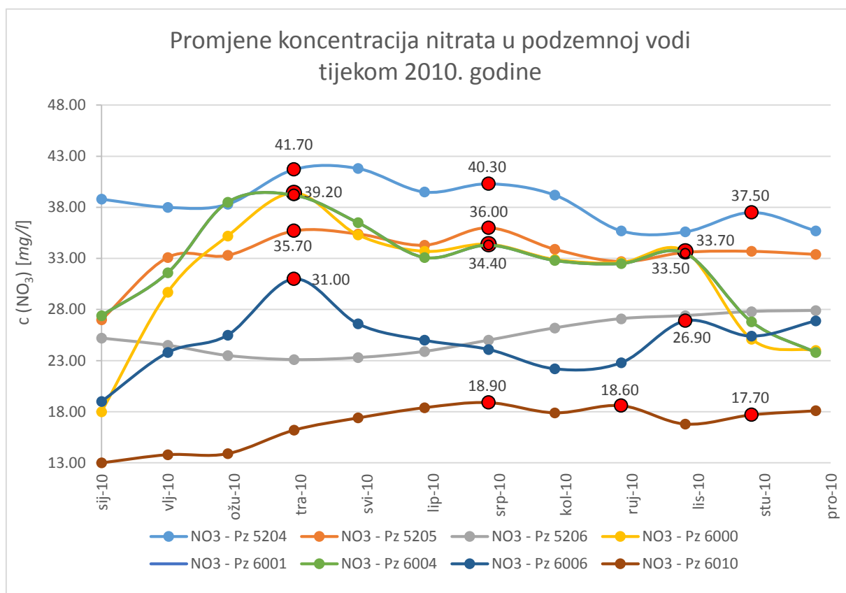
Slika 6.3.4. Mjesečne koncentracije nitrata u podzemnoj vodi u 2010. godini iz 8 piezometara unutar istraživanih područja s naznačenim povišenim vrijednostima koncentracija nitrata
