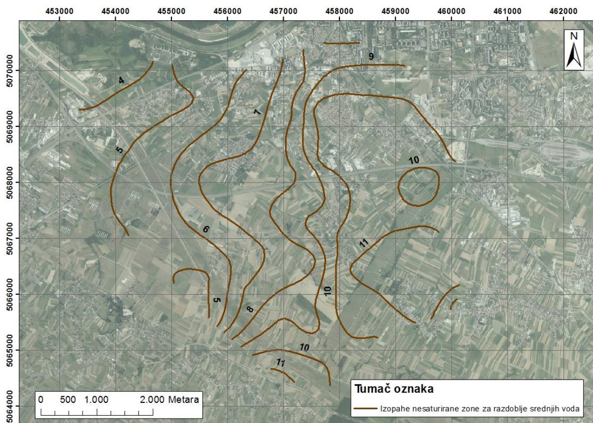
Slika 6.2.7. Karta izopaha nesaturirane zone za razdoblje srednjih voda ( 27.12.2012.) istraživanog područja
