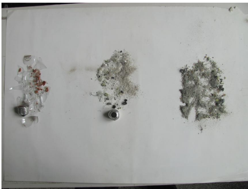
Slika 5-1. Žarulja nakon drobljenja u čeljusnoj, udarnoj i drobilici čekićari (s lijeva nadesno)
