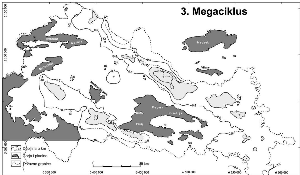
Slika 4-4. Karta izopaha, treći megaciklus (SAFTIĆ et al., 2003)
