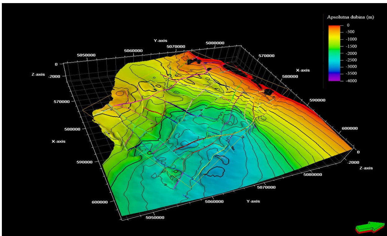
Slika 6-4 Ploha izrađena po EK - markeru Rs5
