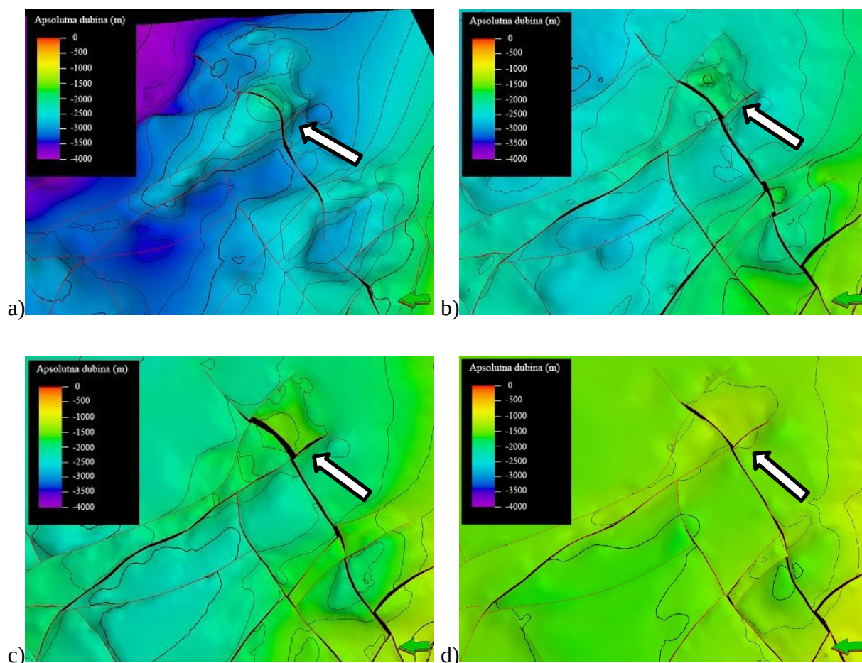
Slika 6-9. Prikaz strukture Veleševac po plohama EK-repera i markera: a) Tg , b) Rs5 , c) Z' , d) Rφ
