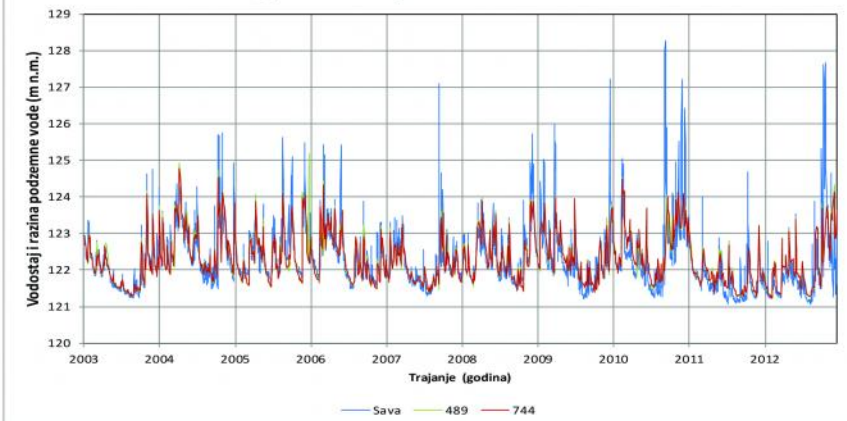
Nivogram Save i piezometara 2003.-2012.
