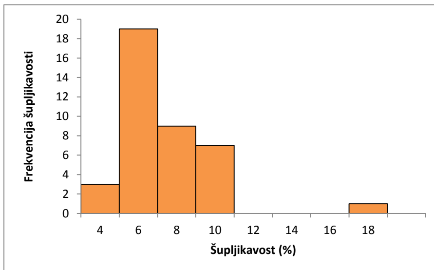
Slika 5-2. Histogram šupljikavosti lapora (krovine) iz bušotine Ša-1 (podatci iz tablice 5-2 )
