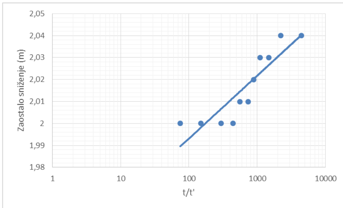
Slika 3.5. Dijagram zaostalog sniženja u piezometru D-1
