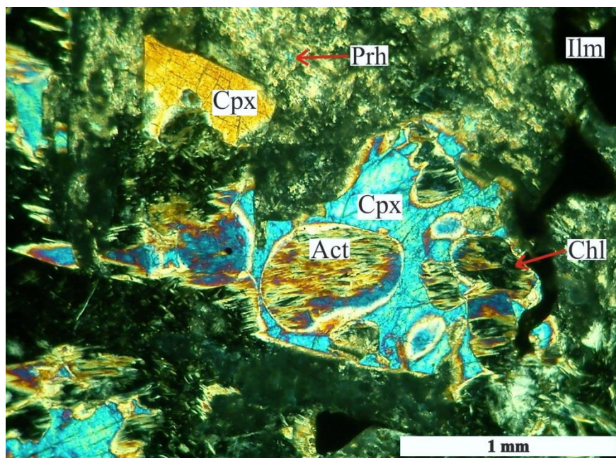
Slika 6-26. Mikrofotografija dijabaza (uzorak RL-5 s lokaliteta Radlovac; N+). Alteracija klinopiroksena u aktinolit i klorit. Act-aktinolit; Chl-klorit; Cpx-klinopiroksen; Ilm-ilmenit; Prh-prehnit.
