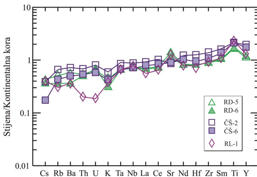
Slika 7-9. Spider dijagram bazičnih i metabazičnih stijena Radlovačkog kompleksa. Koncentracije elemenata u tragovima normalizirane su na prosječni sastav kontinentalne kore. Normalizacijske vrijednosti preuzete su od Rudnick & Gao (2004). Uzorak RL-6, koji zbog naknadne metasomatske promjene ima niže koncentracije Cs, Rb, Ba i K, nije prikazan na dijagramu.
