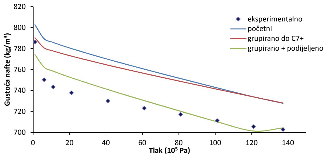
Slika 8-10 Gustoća nafte dobivena eksperimentalno iz DL testa te izračunat Peng-Robinsonovom jednačbom stanja za početni sastav, grupiran do C7+ frakcije te grupiran do C7+ i nakon toga podijeljen
