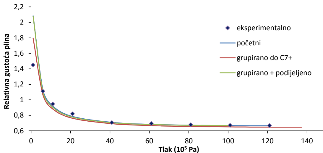
Slika 8-11 Relativna gustoća plina dobivena eksperimentalno iz DL testa te izračunata 3-parametarskom Peng-Robinsonovom jednačbom stanja za početni sastav, grupiran do C7+ i grupiran do C7+ i nakon toga podijeljen
