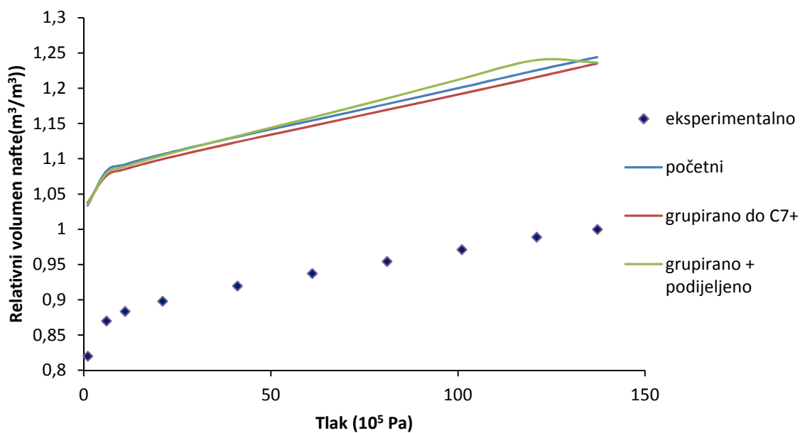
Slika 8-13 Relativni volumen nafte dobiven DL eksperimentom te izračunat Schmidt-Wenzel-ovom jednačbom stanja za početni sastav, grupirano do C7+ frakcije te grupirano do C7+ i nakon toga podijeljen
