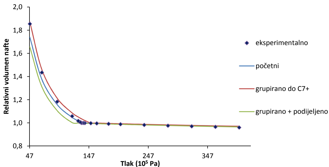
Slika 8-12 Relativni volumen nafte dobiven CCE eksperimentom te izračunat Schmidt-Wenzel-ovom jednačbom stanja za početni sastav, grupirano do C7+ frakcije te grupirano do C7+ i nakon toga podijeljen
