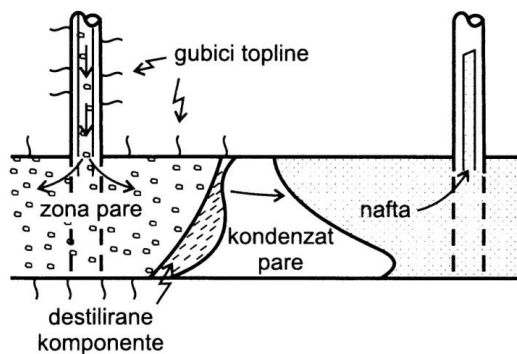
Slika 3-6 Zone zasićenja fluidima pri kontinuiranom utiskivanju pare (Sečen, 2006)
