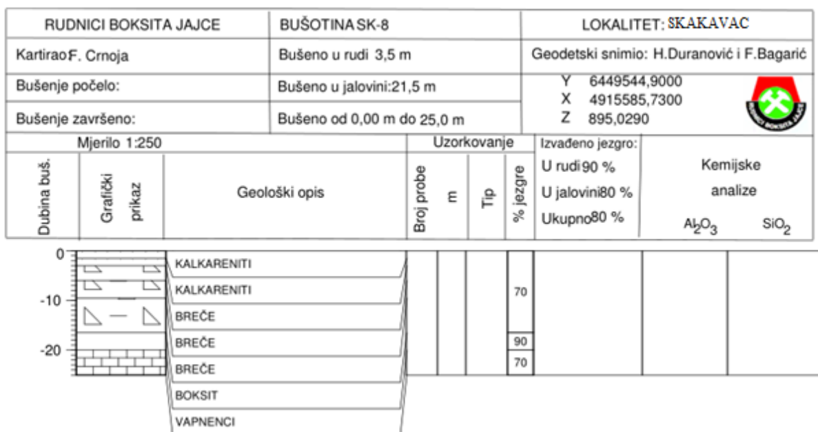
Slika 6-9. Prikaz litološkog stupa bušotine SK8
