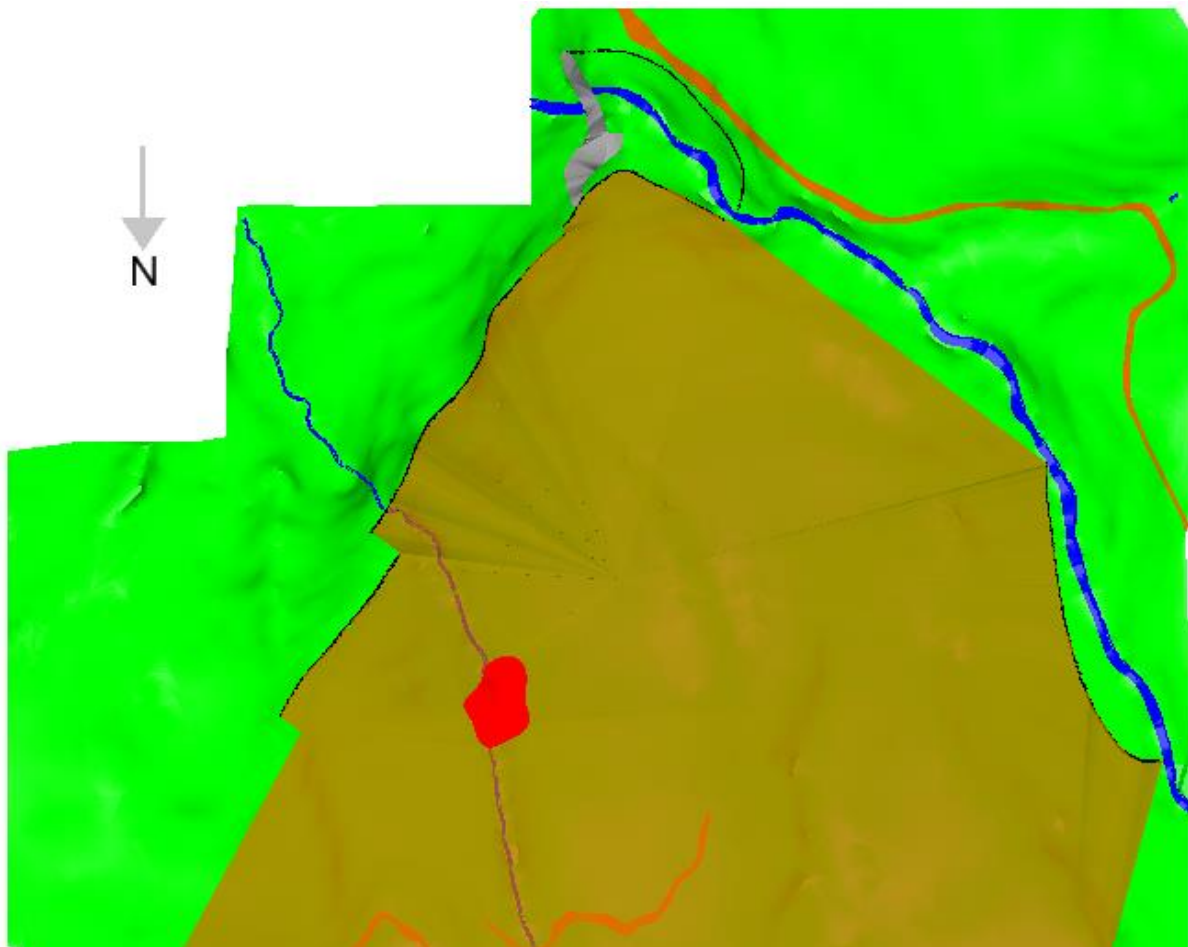
Slika 6-12. Renderirani prikaz površine terena, kontaktne plohe i ležišta boksita na lokalitetu Skakavac
