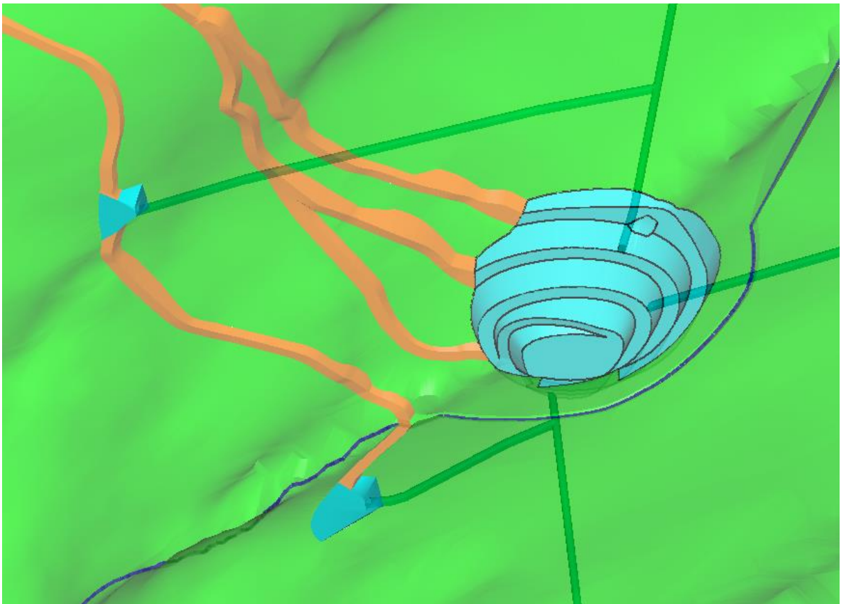
Slika 7-4. Renderirani prikaz većeg površinskog kopa i njegovih pristupnih cesta, te istražnih hodnika
