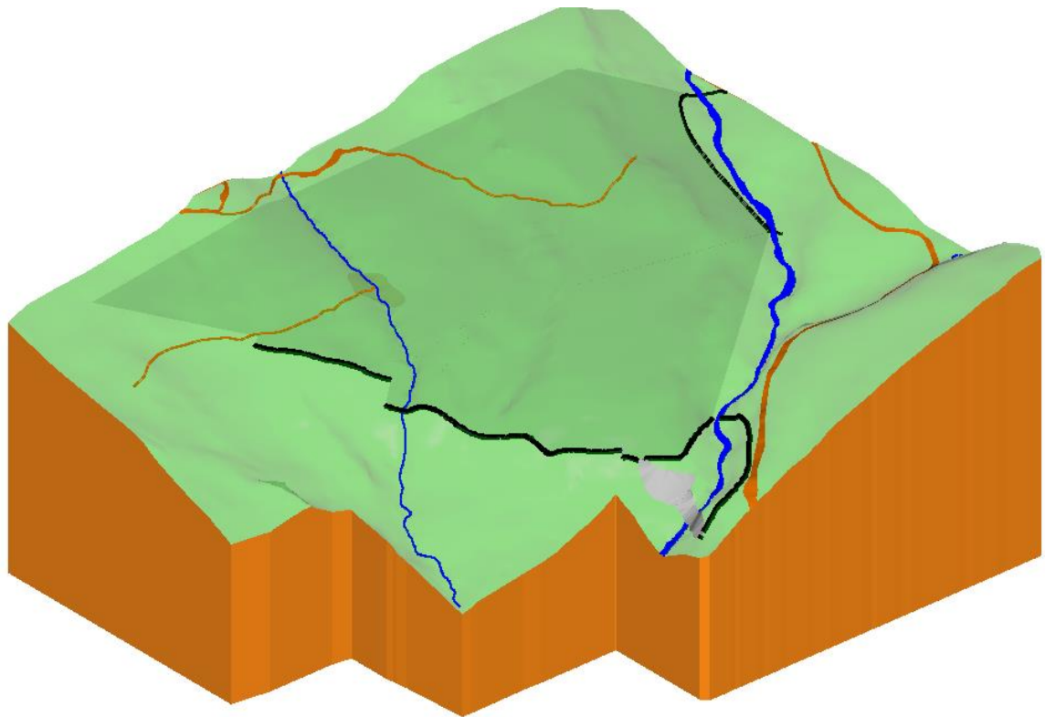
Slika 5-5. Renderirani prikaz terena i kontaktne plohe na lokalitetu Skakavac
