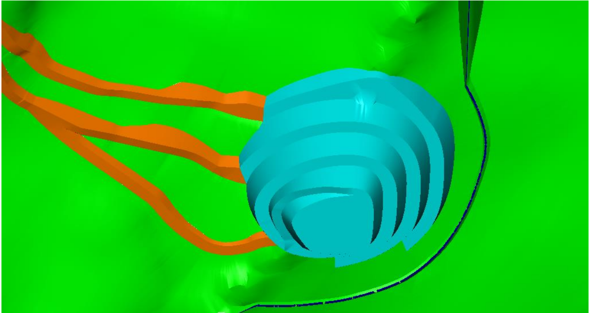
Slika 6-21. Renderirani prikaz većeg kopa i pristupnih cesti za etaže
