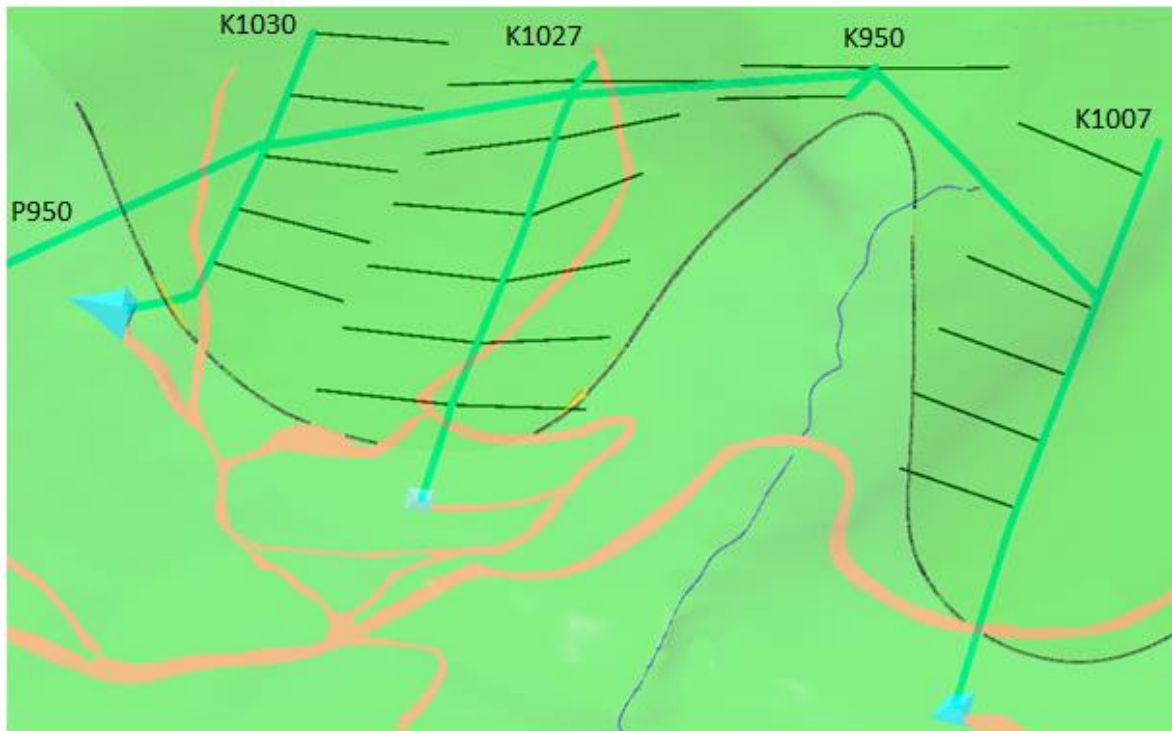
Slika 7-9. Renderirani prikaz površine terena, kontaktne plohe i istražnih radova između lokaliteta Skakavac i Crvene Stijene
