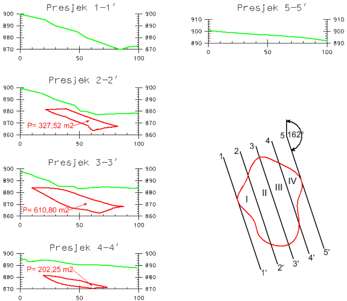
Slika 6-14. Obračunski presjeci modeliranog ležišta boksita, M1:2000
