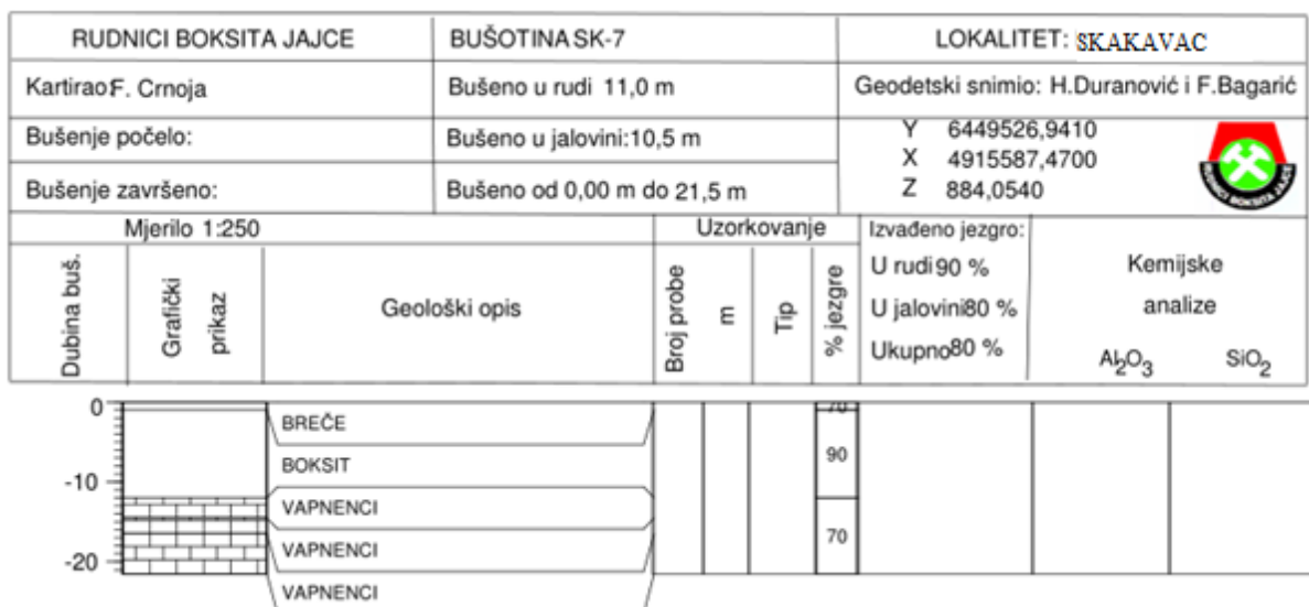
Slika 6-8. Prikaz litološkog stupa bušotine SK7
