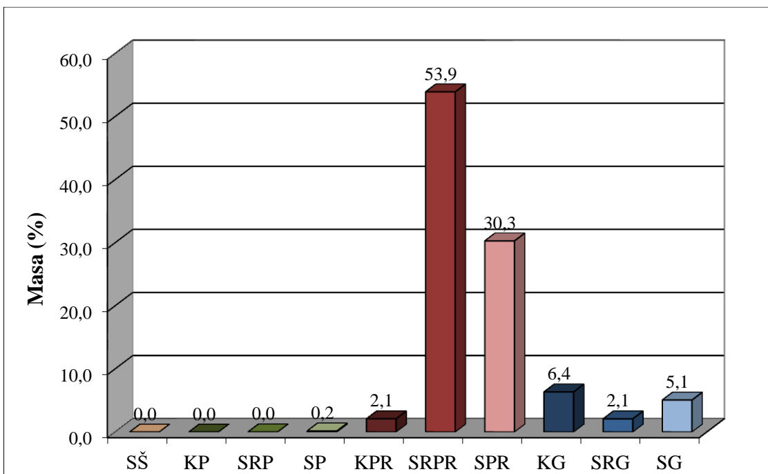
Pirlog 6.2. Histogram granulometrijskih frakcija ( Tumač oznaka: SŠ – sitni šljunak; KP – krupni pijesak; SRP – srednji pijesak; SP – sitni pijesak; KPR – krupni prah; SRPR – srednji prah; SPR – sitni prah; KG – krupna glina; SRG – srednja glina; SG – sitna glina ).
