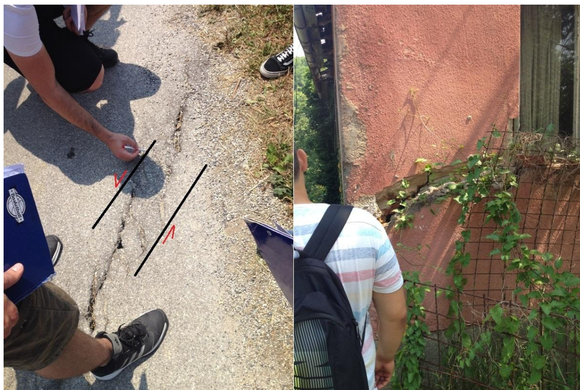
Slika 3.1. Oštećenja kao pokazatelji utjecaja klizišta Kostanjek (lijevo: vlačna pukotina na asfaltiranoj javnoj prometnici; desno: šteta na privatnom vlasništvu).
