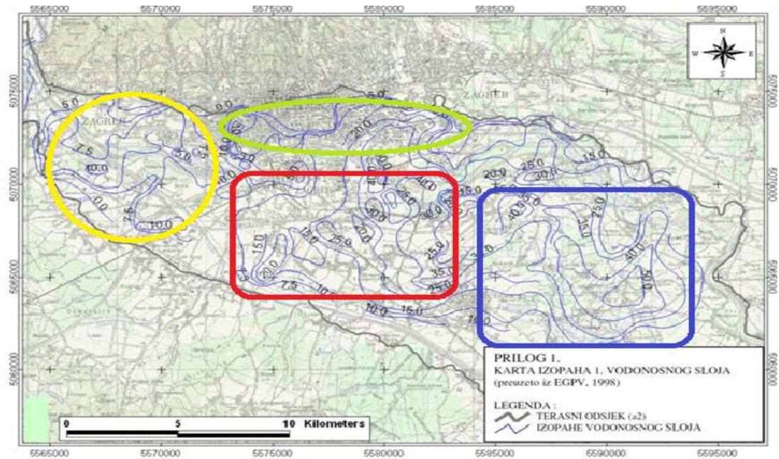
Slika 3.5. Izopahe aluvija (Miletić i Bačani, 1999)
