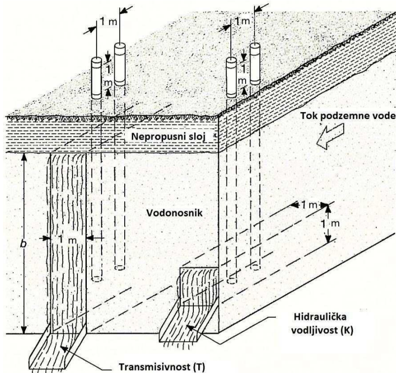
Slika 2.3. Hidraulička vodljivost (Driscoll, 1986)
