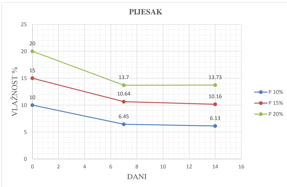
Slika 5-4. Odnos vlažnosti i vremena kod pijeska
