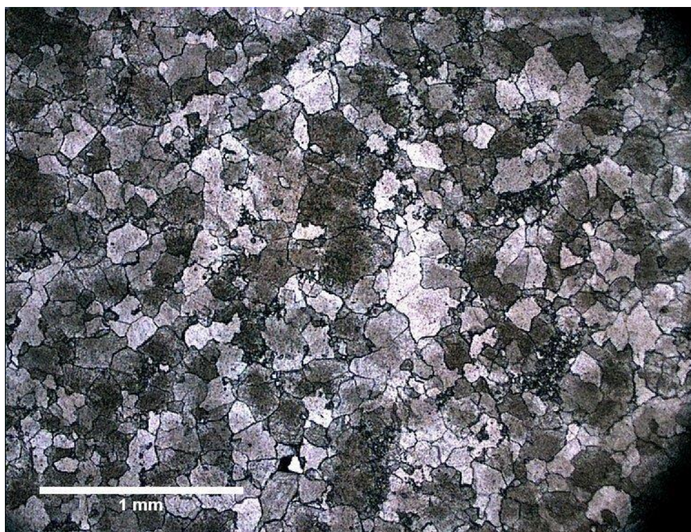
Slika 6.7. Mikrofotografija uzorka G-6 – struktura kasnodijagenetskog dolomita
