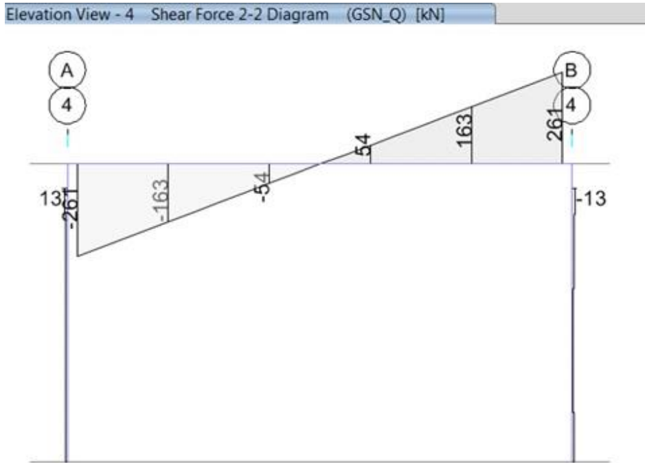
Slika 6-13. Dijagram poprečnih sila - vertikalno opterećenje
