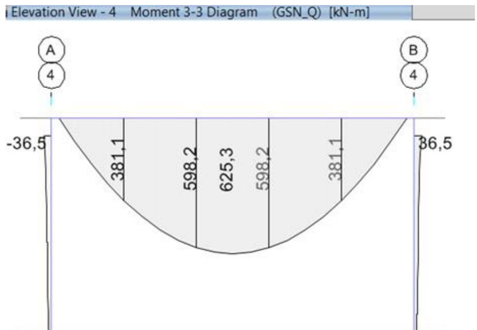
Slika 6-14. Dijagram momenta savijanja - vertikalno opterećenje
