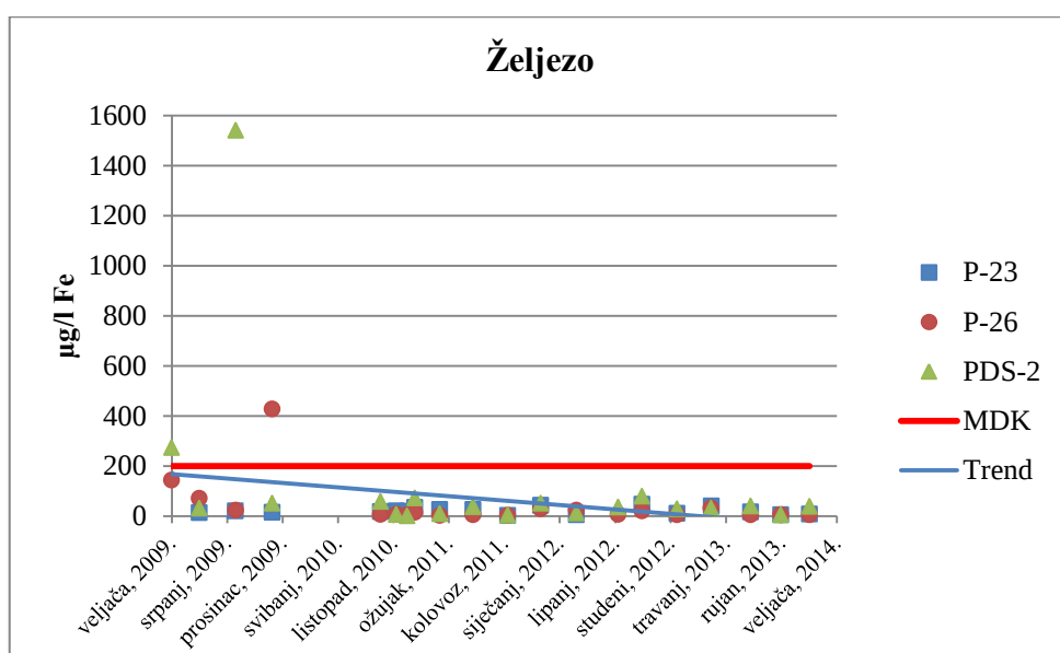
Slika 4.13. Željezo u podzemnoj vodi priljevnom području crpilišta Nedelišće
