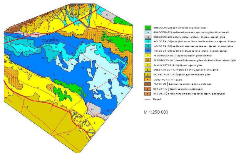
Slika 2-2. Geološka karta grada Zagreba i Zagrebačke županije (Bačani i Šparica, 2001)
