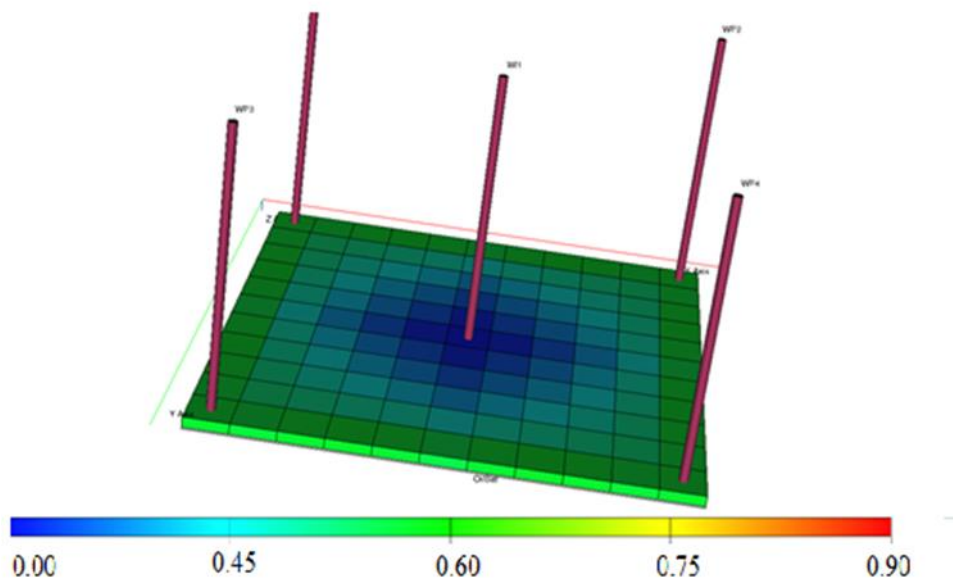
Slika 7-12. Zasićenje naftom na kraju trećeg perioda
