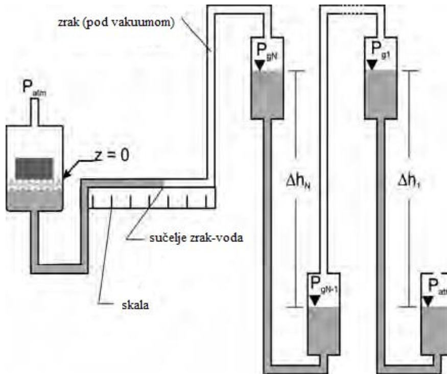
Slika 4-6. Metoda višestrukih negativnih stupaca vode (Tarantino i dr., 2008).
