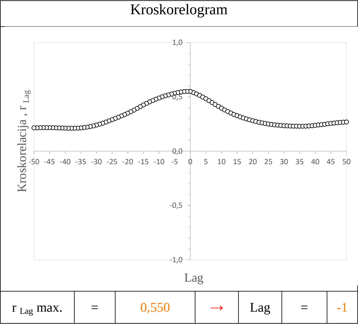
Slika 5-3. Kroskorelogram
