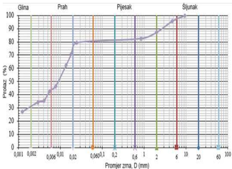
Slika 5-8 Granulometrijska krivulja
