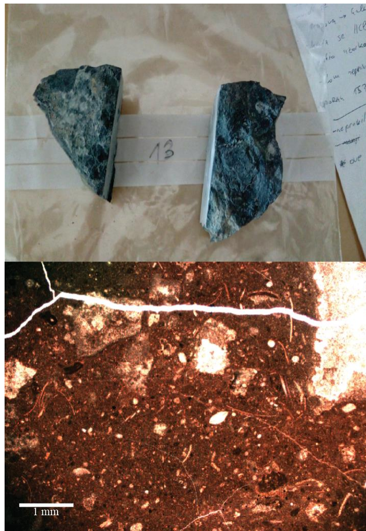
Slika 6.7. Uzorak iz sloja 13 makroskopski uzorak (gore), te veliki broj raznih alokema u mikroskopskom preparatu (dolje).
