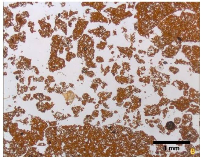
Slika 5 – 21. Pedalitet preparat 2: A(-) i B(+): djelovi preparata 2 s poliedričnim granulama kao agregatima
