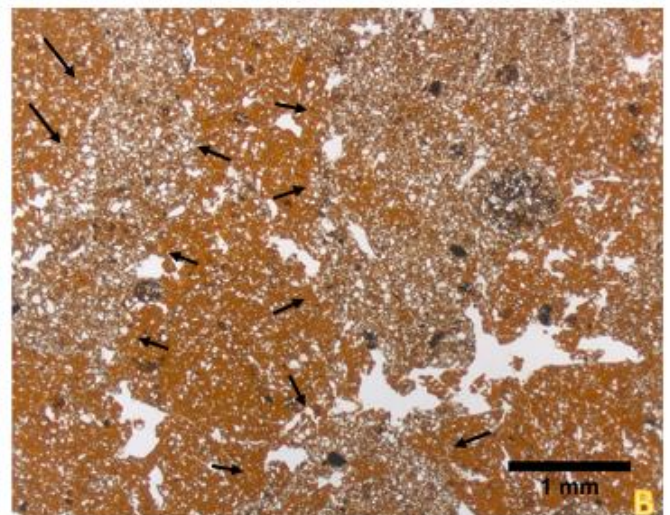
Slika 5 – 22. A(-) i B(-): strelicama označene matriks pedotvoreine
