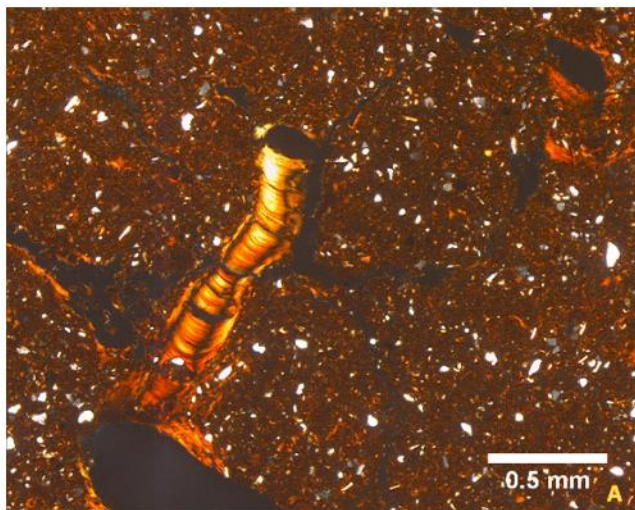
Slika 5 – 59. A(-): martiks pedotvorenina (impregnativna pedotvorenina) – srpasta glinovita prevlaka i srpastostrijasti tip građe mikromase, oko kojega se nalazi točkasto - pjegasti tip b-građe i otvorena porfirna c/f distribucija; B(-): inrtuzivna pedotvorenina – anortična impregnirana nodula
