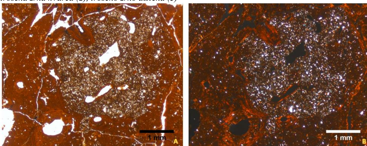
Slika 5 – 57. Matriks pedotvorenina; A(-): impregnativna pedotvorenina; B(+): krupnozrnati mineralna frakcija unutar impregnativne pedotvorenina za razliku od ostatka matriksa
