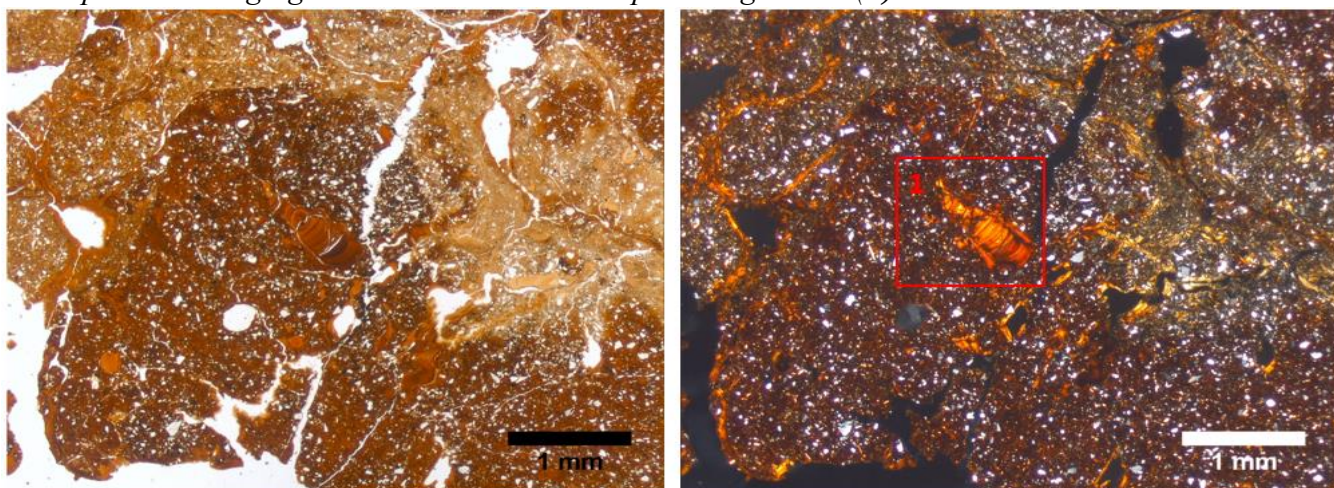
Slika 5 – 52. Matriks pedotvorevine A(-): dio preparata zahvaćen procesom ožučivanja, narančasto – žute boje i klastične glinovite prevlaka u donjem lijevom dijelu prepata; B(+): točkasto - pjegasti i porostrijasti tip b – građe; srpasta glinovita prevlaka nastala unutar vagova (1)
