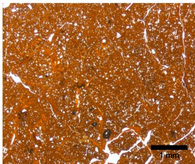
Slika 5 – 45. Tip građe mikromase preparat 5: A(+) i B(-):unakrnostrijasti tip b-građe mikromase
