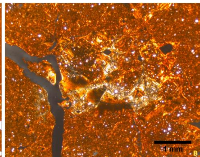
Slika 5 – 62. A(-) i B(-) Nakupina glinovitih tipičnih i srpaste glinovitih prevlaka u preparatu, pojedini dijelovi svijetlije su obojeni jer su zahvaćeni procesom ožučivanja
