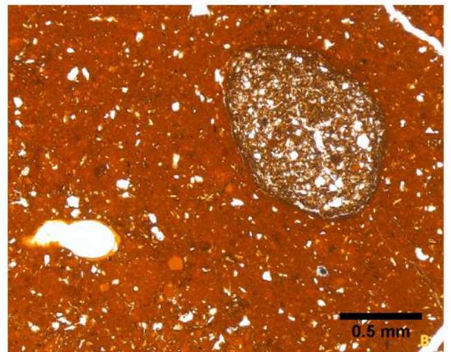
Slika 5 – 59. A(-): martiks pedotvorenina (impregnativna pedotvorenina) – srpasta glinovita prevlaka i srpastostrijasti tip građe mikromase, oko kojega se nalazi točkasto - pjegasti tip b-građe i otvorena porfirna c/f distribucija; B(-): inrtuzivna pedotvorenina – anortična impregnirana nodula
