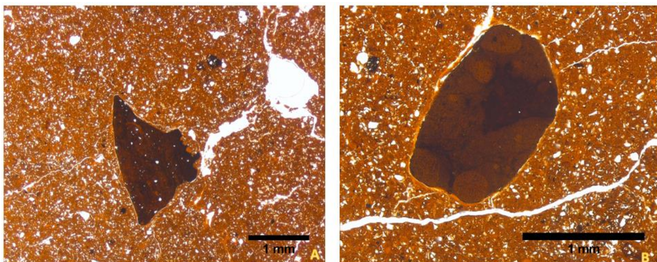
Slika 5 – 42. intruzivne pedotvorenine; A(-): pedorelikt nepravilnog oblika, B(-): litorelikt (boksit) s vidljivim obrubom glinovitih prevlaka
