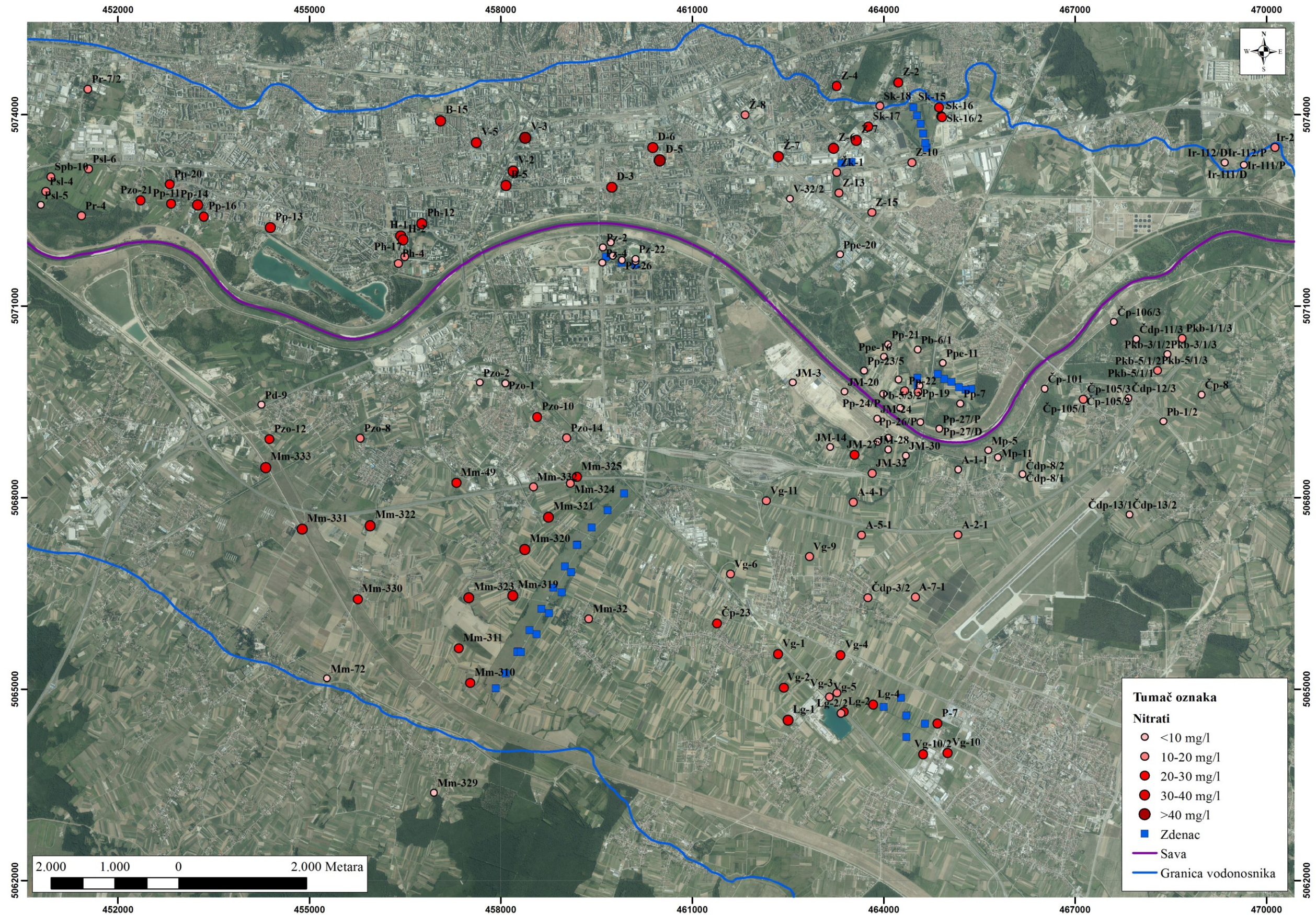
Slika 6.4. Prosječne koncentracije nitrata u zagrebačkom vodnosniku u razdoblju od 1991. do 2015. godine (modificirano prema Kovač et al., 2017a)
