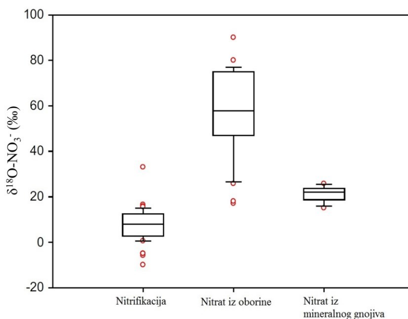
Slika 4.7. Dijagram pravokutnika koji prikazuje \delta^{18}\text{O}-\text{NO}_3^- nastalog putem nitrifikacije, iz oborina i iz mineralnog gnojiva (Xue et al., 2009)
