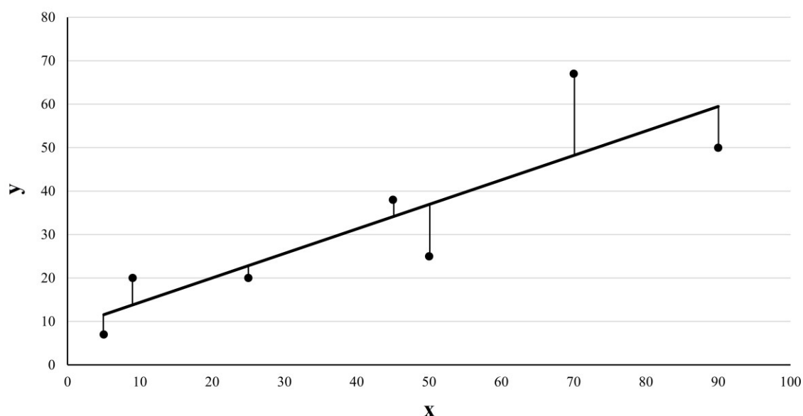
Slika 4.25. Prikaz reziduala u regresiji
