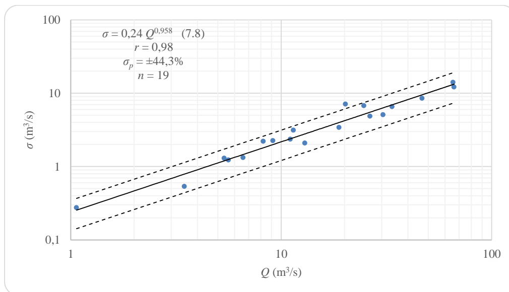
Slika 7.7 Nelinearna ovisnost standardne devijacije srednjih godišnjih protoka \sigma o srednjim godišnjim protocima Q s intervalom pouzdanosti \sigma_p izvedene s 19 podataka
