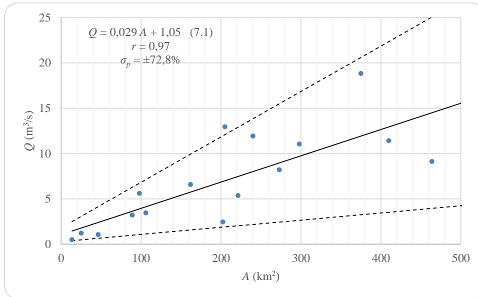
Slika 7.3 Linearna ovisnost srednjih godišnjih protoka Q o površini slivova A s intervalom pouzdanosti \sigma_p u području slivnih površina do A = 500 \text{ km}^2
