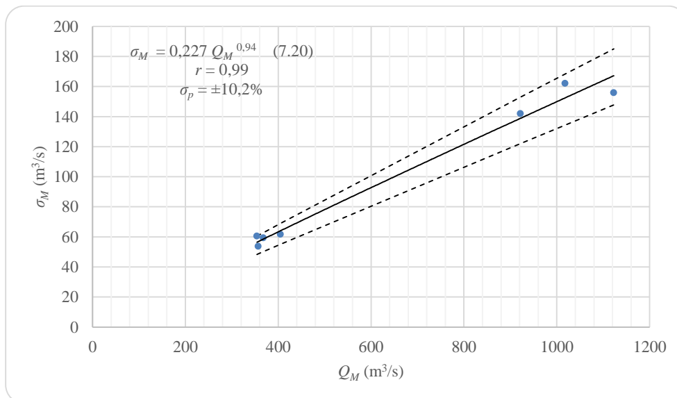
Slika 7.11 Linearna ovisnost standardne devijacije maksimalnih zabilježenih godišnjih protoka \sigma_M o maksimalnim zabilježenim godišnjim protocima Q_M s intervalom pouzdanosti \sigma_p izvedene sa 7 podataka
