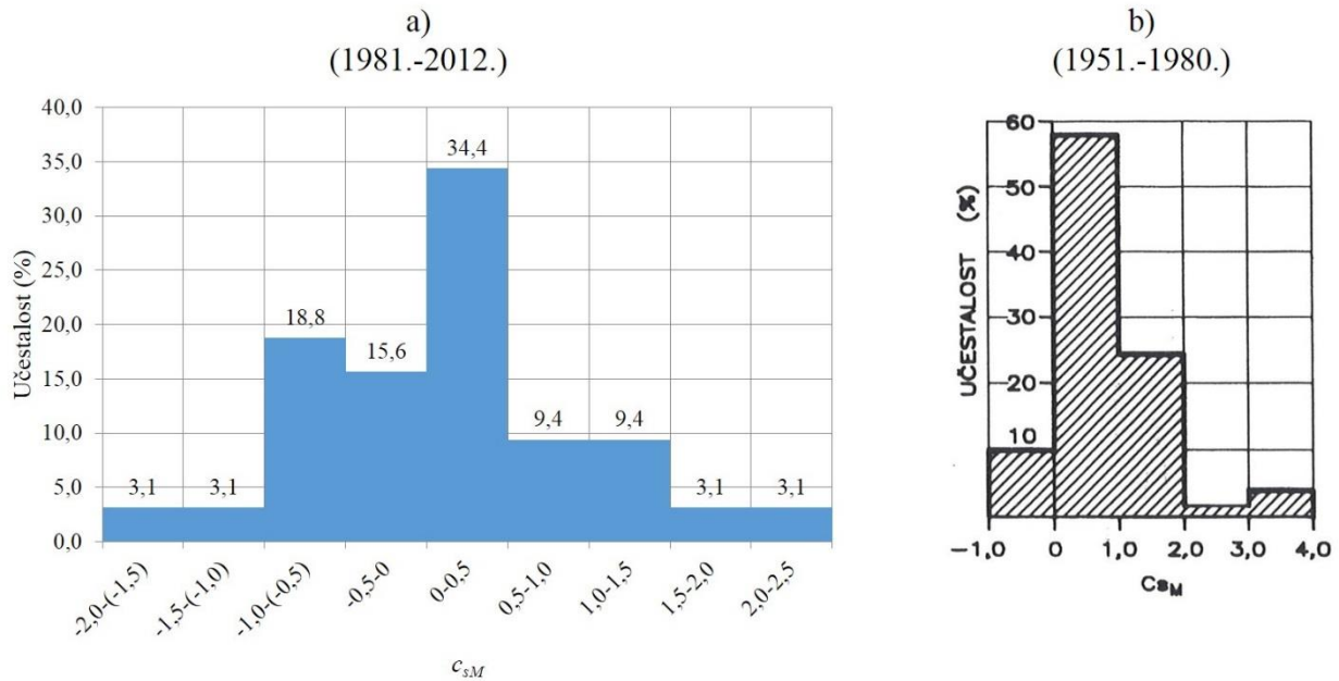
Slika 6.11 Histogram učestalosti koeficijenta asimetrije maksimalnih godišnjih protoka c_{sM} a) za razdoblje obrade (1981.-2012.), b) prema ranijoj obradi hrvatskog krša iz 1995. godine
