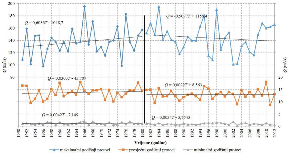
Slika 5.7 Maksimalni, srednji i minimalni godišnji protoci Kupe u profilu Kupari u razdobljima (1951.-1980.) i (1981.-2012.)
