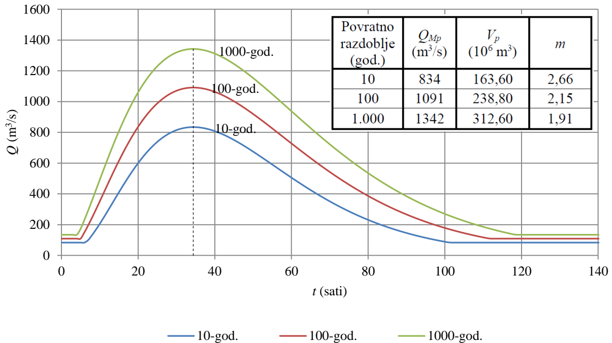
Slika 7.22 Vodni valovi 10-, 100- i 1000-godišnjeg povratnog razdoblja na profilu Radenci na rijeci Kupi. Vrijeme podizanja vodnih valova je 34,4 sata a ukupno trajanje vodnih valova je 138 sati.
