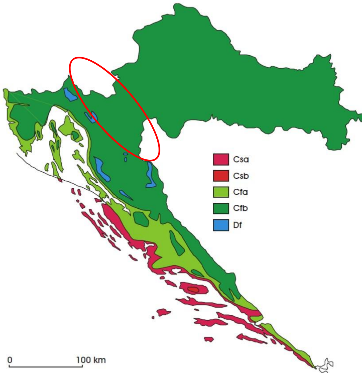
Slika 3.10 Geografska raspodjela klimatskih tipova po W. Köppenu u Hrvatskoj u standardnom razdoblju (1961.-1990.): Cfa, umjereno topla vlažna klima s vrućim ljetom; Cfb, umjereno topla vlažna klima s toplim ljetom; Csa, sredozemna klima s vrućim ljetom; Csb, sredozemna klima s toplim ljetom; Df, vlažna borealna klima; crvenom elipsom je označeno područje istraživanja (preuzeto iz Šegota i Filipčić, 2003)
