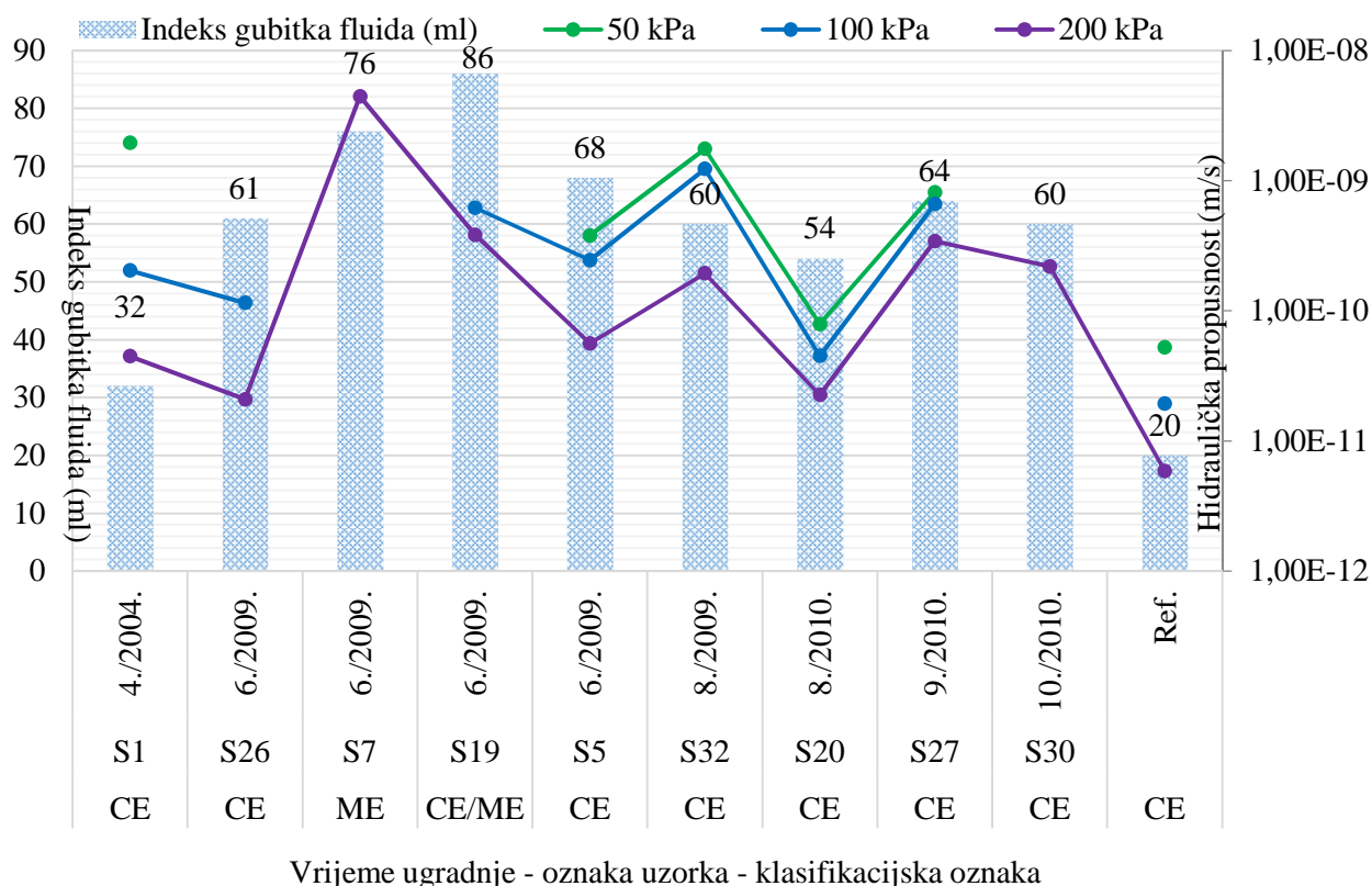
Slika 12-10 Prikaz zavisnosti hidrauličke propusnosti o indeksu gubitka fluida i efektivnim konsolidacijskim napreznjima
