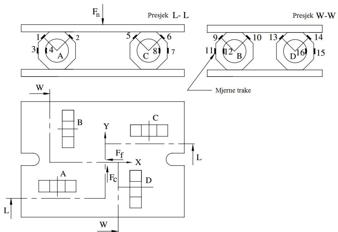
Slika 6.6. Položaj tenzometarskih traka i prstena na mjernom pretvorniku sile (Yaldız i Ünsaçar, 2006).
