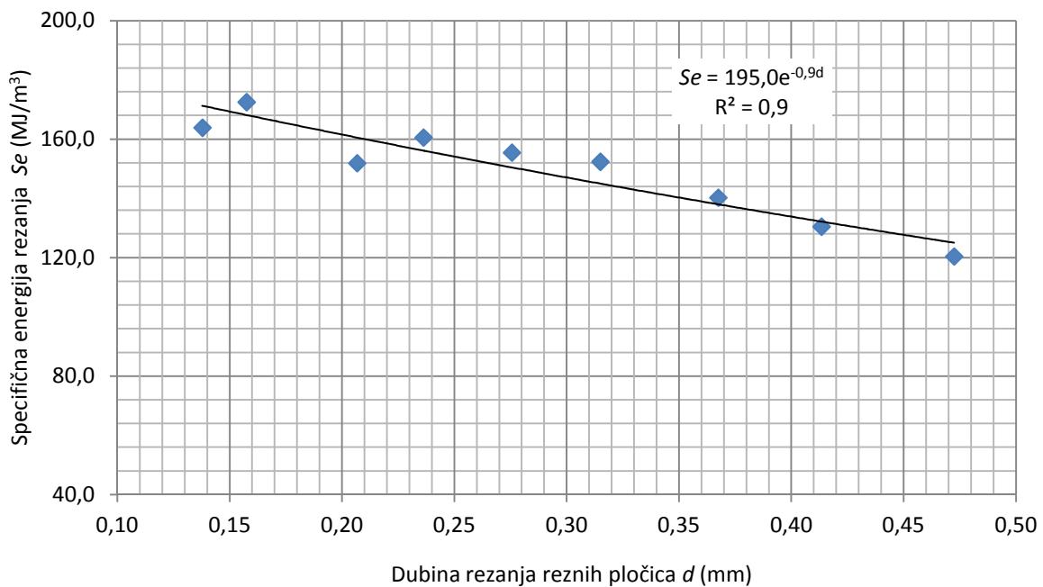
Slika 6.39. Zavisnost specifične energije rezanja i dubine rezanja rezne pločice.
