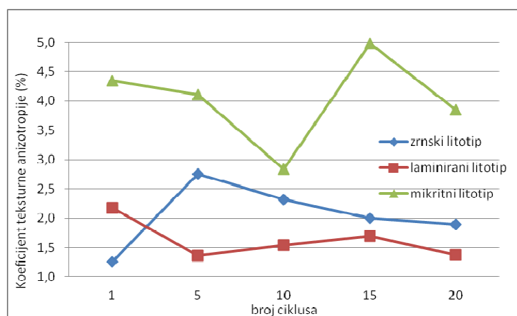
SI.5.53. Promjena koeficijenta teksturne anizotropije (%) uzoraka tijekom 20 ciklusa toplinske promjene.
