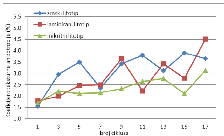
SI.5.51. Promjena koeficijenta teksturne anizotropije (%) uzoraka tijekom 15 ciklusa kristalizacije soli.
