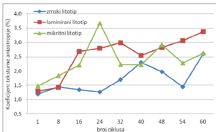
SI.5.52. Promjena koeficijenta teksturne anizotropije (%) uzoraka tijekom 55 ciklusa smrzavanja.
