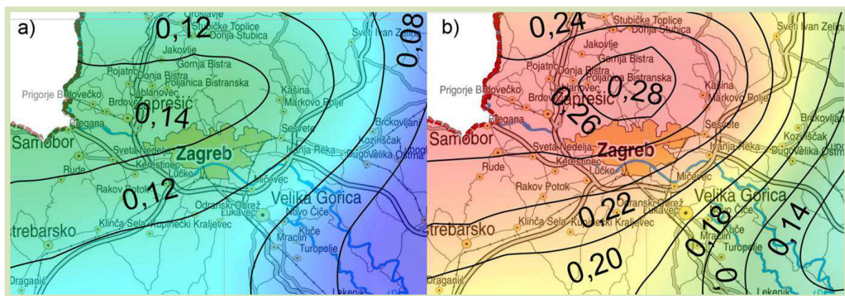
Slika 8 Izsečki Karte potresnih područja Republike Hrvatske za poredbena vršna ubrzanja temeljnog tla tipa A ( Herak, 2011a; 2011b ): a) s vjerojatnosti premašaja 10% u 10 godina, za povratno razdoblje 95 godina u jedinicama gravitacijskog ubrzanja g; b) s vjerojatnosti premašaja 10% u 50 godina, za povratno razdoblje 475 godina u jedinicama gravitacijskog ubrzanja g
