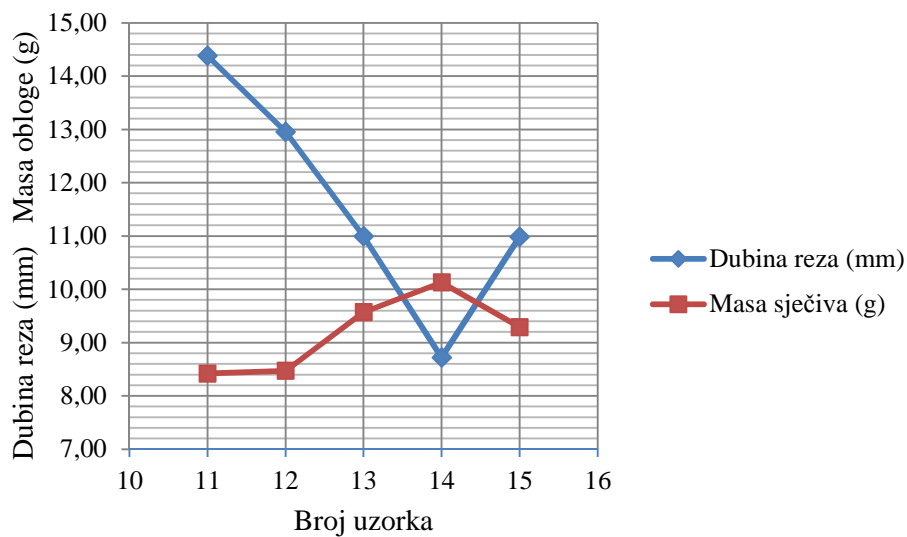
Slika 6-84. Odnos mase sječiva i dubine reza za Al-metu, 10% čeličnog praha
