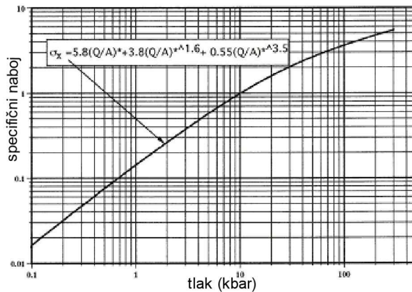
Slika 6-37. Mjerni dijagram za očitavanje tlaka
