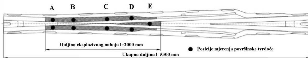
Slika 3-15. Pozicije mjerenja tvrdoće materijala (Havliček & Nesvadba 2011)
