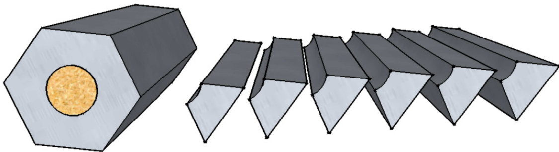
Slika 3-8. Fragmentacija šesterokutne prizme s provrtom napunjenim eksplozivom
