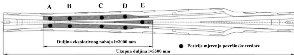
Slika 3-15. Pozicije mjerenja tvrdoće materijala (Havliček & Nesvadba 2011)
