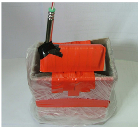
Slika 6-20. Ispitivanje oblika i stanja obloge –postav II u vodi
