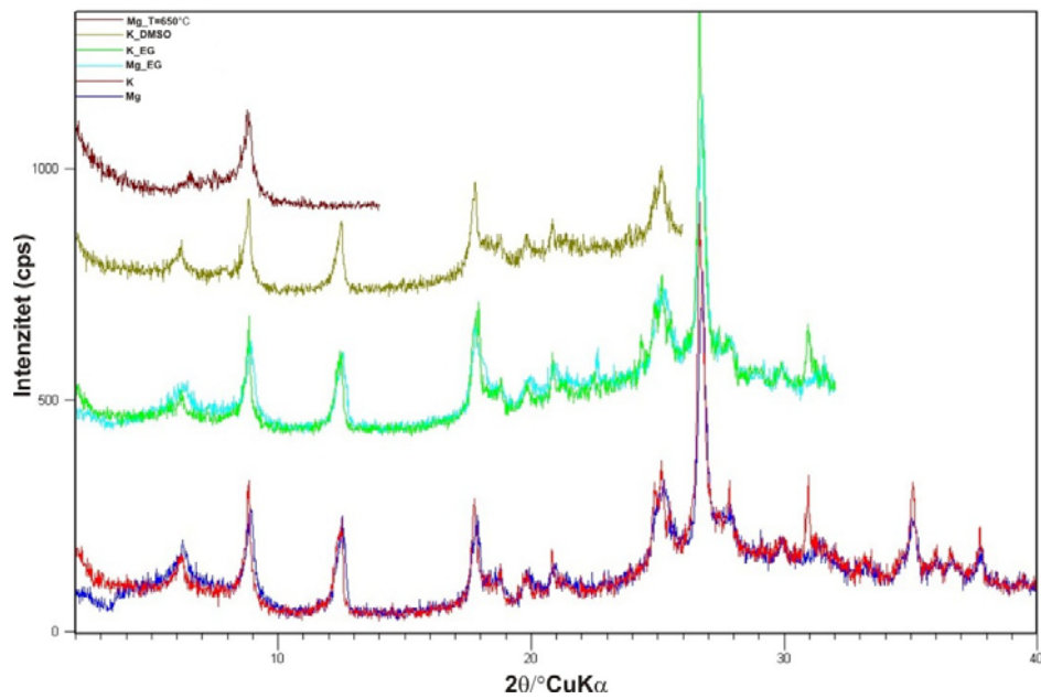
Difrakcijske slike orijentirane frakcije < 2\mu\text{m} IV Gso/Gr horizonta tla s pedološkog profila.
