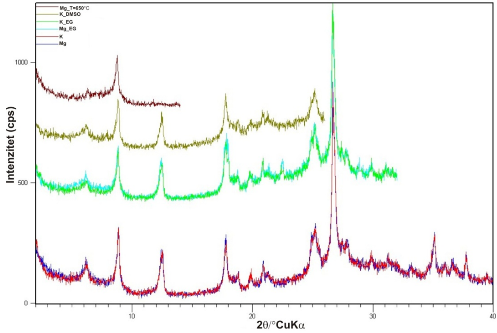
Difrakcijske slike orijentirane frakcije < 2\mu\text{m} III Gso horizonta tla s pedološkog profila.
