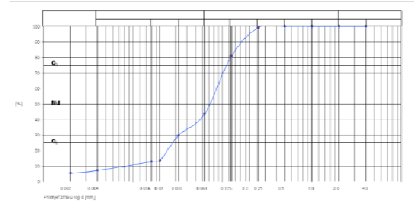
Granulometrijska krivulja za horizont IIIGso
