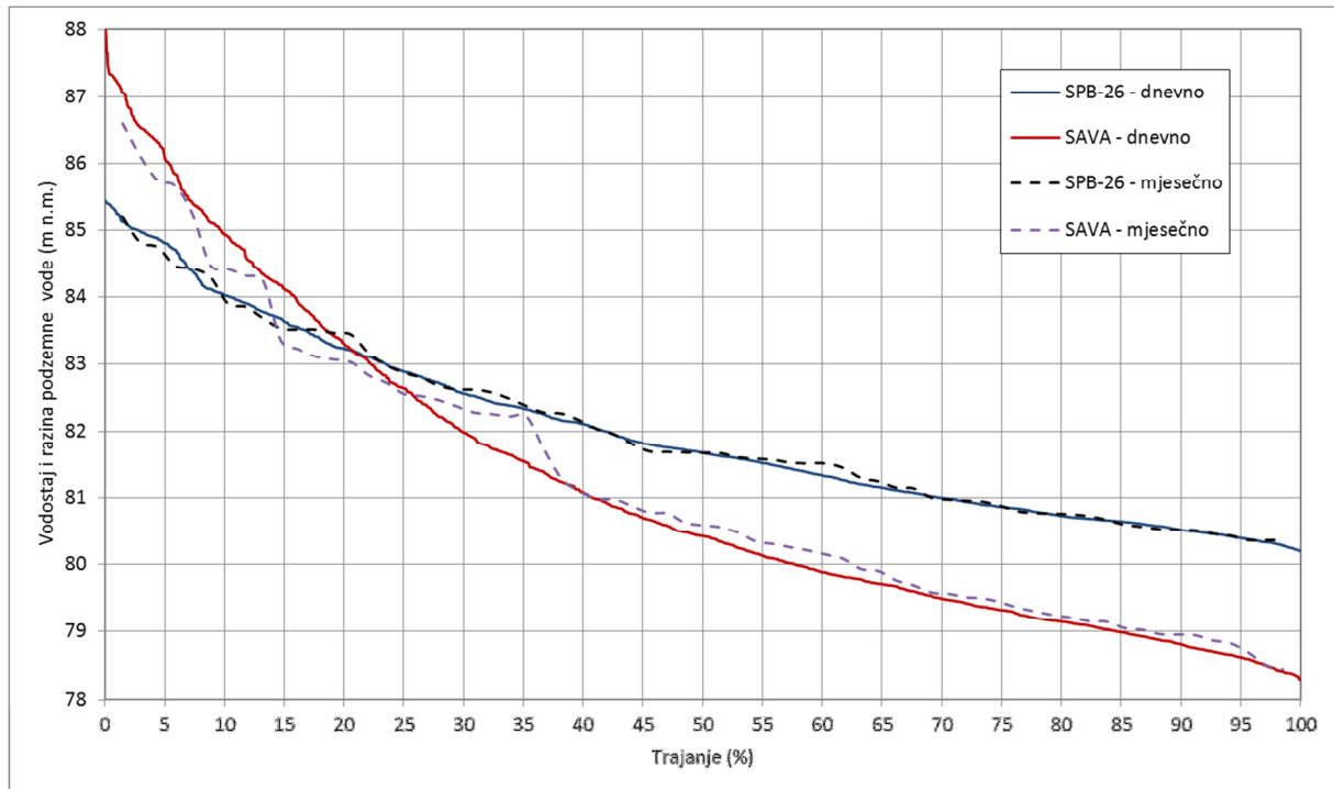
Slika 7.31 Usporedba krivulja trajanja vodostaja rijeke Save i razine podzemne vode s dnevnim i osrednjenim mjesečnim podacima (lipanj 2008 – prosinac 2013)
