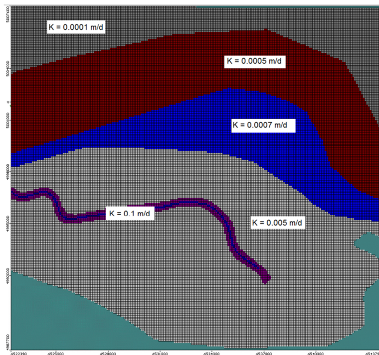
Slika 7.26 Različite zone hidrauličke vodljivosti u krovinskim naslagama
