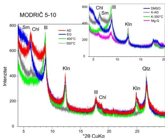
Prilog 75. Rendgenogram orijentiranog preparata uzorka iz jezgre MOD-A. Oznake: AD-sušen na zraku, EG-tretiran s etilen glikolom, G-tretiran s glicerolom, DMSO-dimetil sulfoksidi, Ill-ilit, Kln-neuređen kaolinit, KlnD-uređen kaolinit, V-vermikulit, Qtz-kvarc, I-V-ilit-vermikulit.
