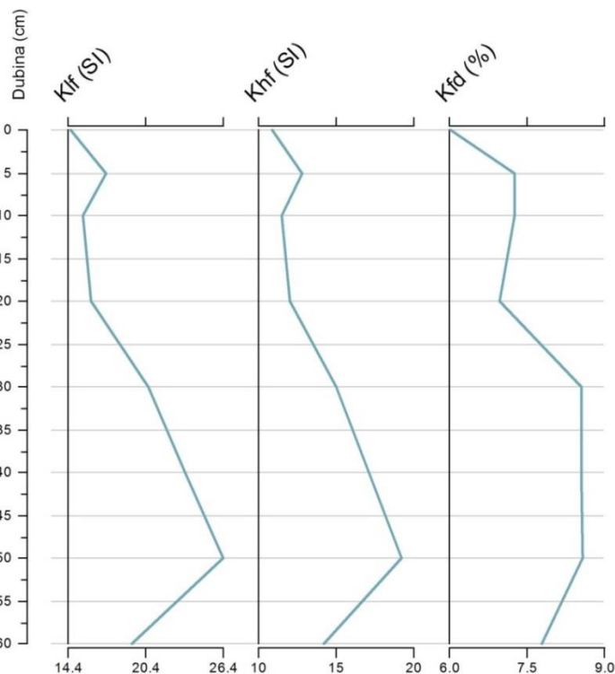
Slika 5.147. Dubinska raspodjela susceptibiliteta na niskoj frekvenciji ( \kappa_{lf} (SI)), visokoj frekvenciji ( \kappa_{hf} (SI)) i razlike susceptibiliteta mjenenog na visokoj i niskoj frekvenciji ( \chi_{fd} %) mjerena senzorom MS2B u jezgri 505/T.
