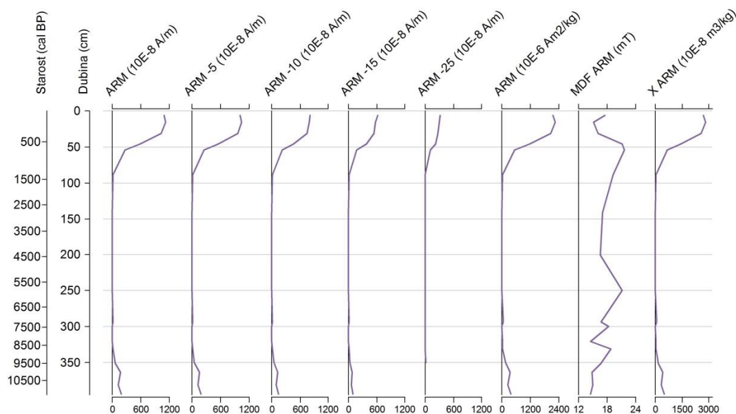
Slika 5.154. Vertikalna raspodjela ARM-a, demagnetizacije ARM-a pri vanjskom magnetskom polju od 5mT do 25mT, \text{MDF}_{\text{ARM}} -a i \chi_{\text{ARM}} u jezgri KAR-A.
