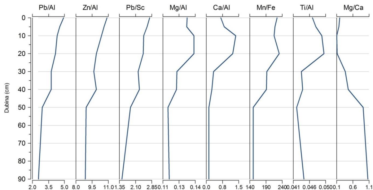
Slika 5.84. Raspodjela odabranih odnosa kemijskih elemenata (Pb/Al, Zn/Al, Pb/Sc, Mg/Al, Ca/Al, Mn/Fe, Ti/Al, Mg/Ca) u jezgri 505T.
