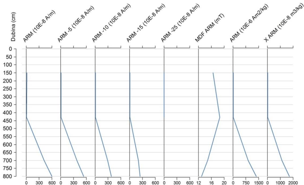
Slika 5.202. Vertikalna raspodjela ARM-a, demagnetizacije ARM-a pri vanjskom magnetskom polju od 5mT do 15mT, MDF ARM -a i \chi_{\text{ARM}} u jezgri NOV-11.
