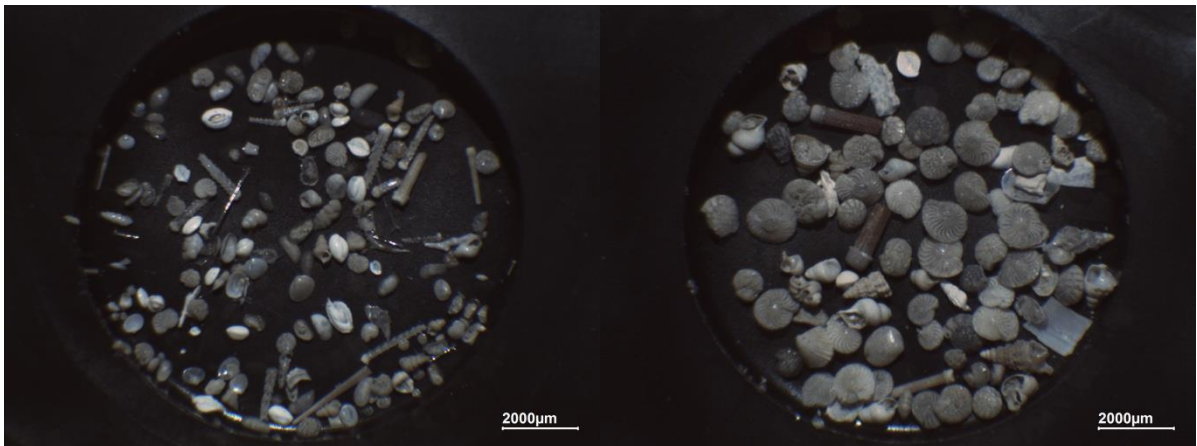
Prilog 117. Fosilni sadržaj uzorka MOD-A 317-320.
