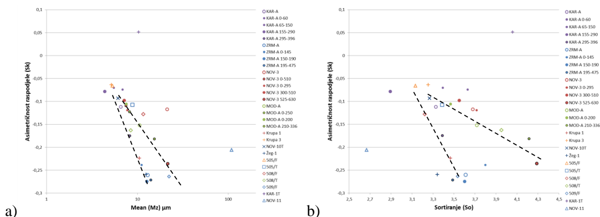
Slika 6.1. a) odnos asimetričnosti raspodjele ( S_k ) i prosječne veličine zrna ( M_z ) u svim uzorcima. Uzorci imaju simetričnu raspodjelu krivulje ukoliko se nalaze u intervalu 0,1 do -0,1; krivulje su pozitivno nakošene za S_k < -0,1 . b) odnos asimetričnosti raspodjele ( S_k ) i sortiranja ( S_o ).
