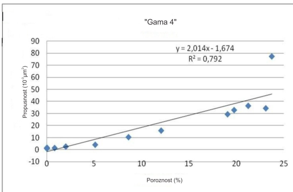
Slika 6-16. Jednadžba krivulje ovisnosti poroznosti i propusnosti za ležište Gama 4
