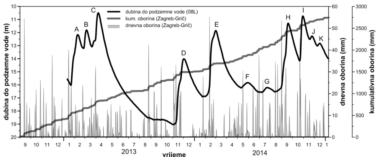
Slika 6.2. Dnevne i kumulativne oborine izmjerene na meteorološkoj postaji Zagreb-Grič te dubine do podzemne vode izmjerene na klizištu Kostanjek, za razdoblje od rujna 2012. do siječnja 2015. godine.
