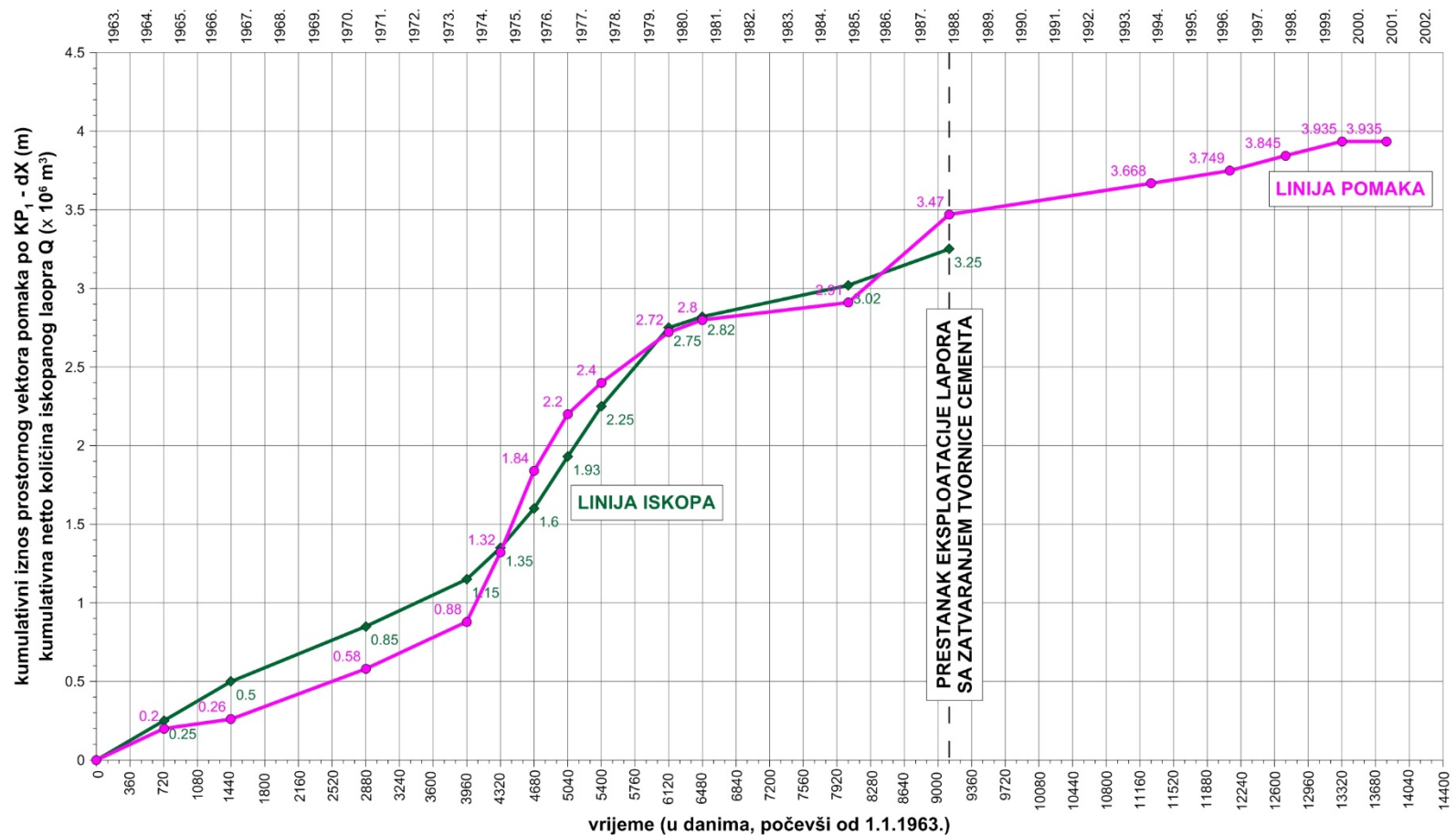
Slika 3.19. Kumulativni prostorni pomaci klizišta Kostanjeek po najdubljoj kliznoj plohi KP1 od početka klizanja 1963. do travnja 2001. godine s kumulativnom neto količinom iskopanog lapora od početka klizanja do prestanka eksploatacije (precrtano iz Ortolan, 2008).
