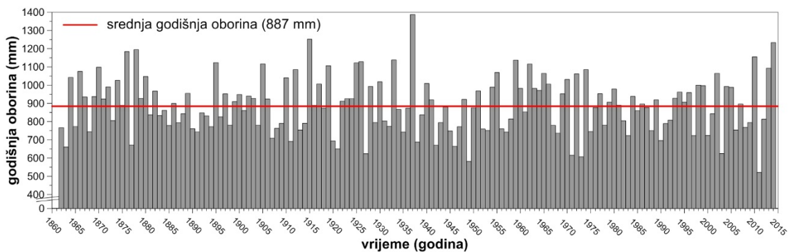
Slika 3.8. Prikaz godišnjih oborina izmjerениh na meteorološkoj postaji Zagreb-Grič za razdoblje od 1862. do 2014. godine.
