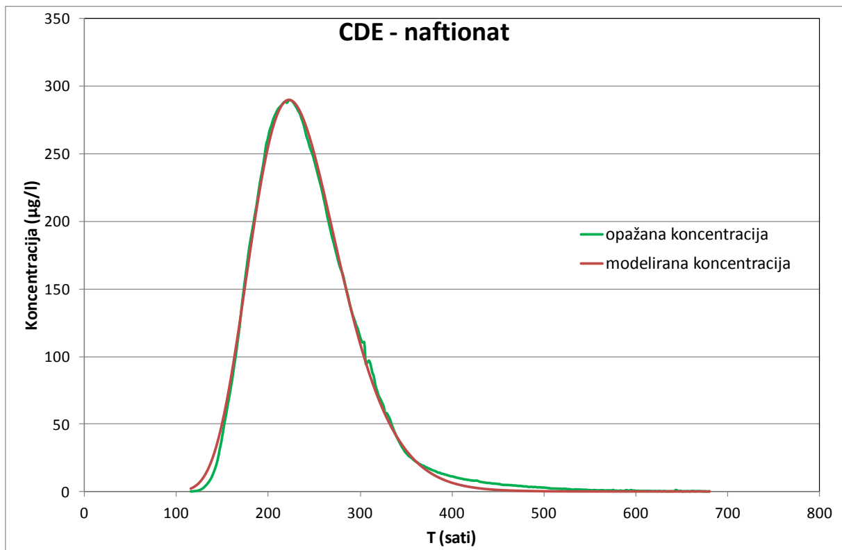
Slika 7.49. Rezultati CDE modela za trasiranje naftionatom izvedeno u lipnju 2012. godine
