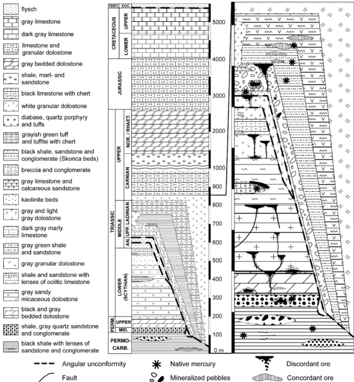
Slika 3.1. Sintetski stratigrafski stup Idrijskog ležišta (preuzeto iz: Lavrič i Spangenberg, 2003)
