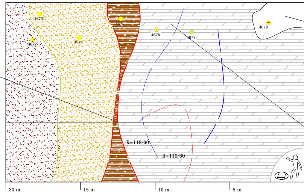
Orudjenje u anizičkom dolomitu, desni bok, 3 m
